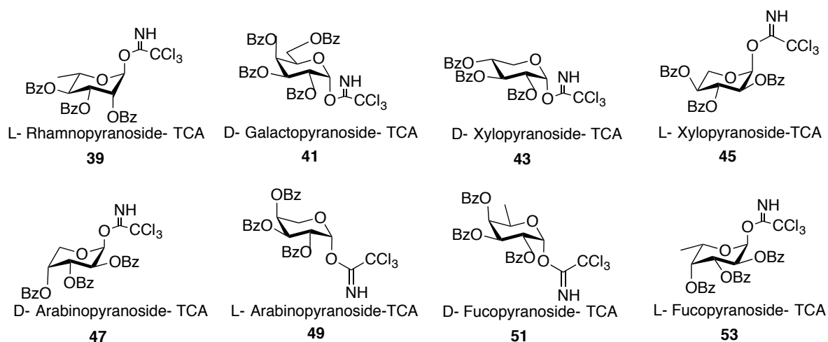
Figure 7 : Liste des saccharides trichloroacétimidates synthétisés
