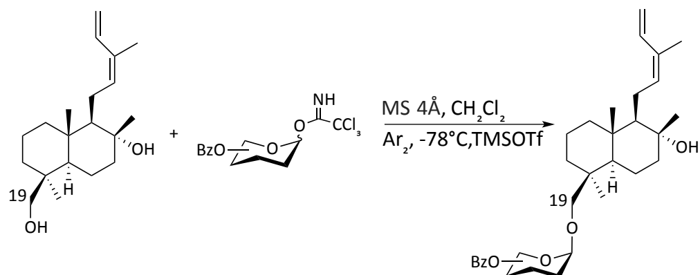
Figure 14 : Glycosylation du 19- cis -hydroxiabiéniol
