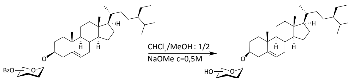
Figure 17 : Déprotection des glycosides du \beta -sitostérol
