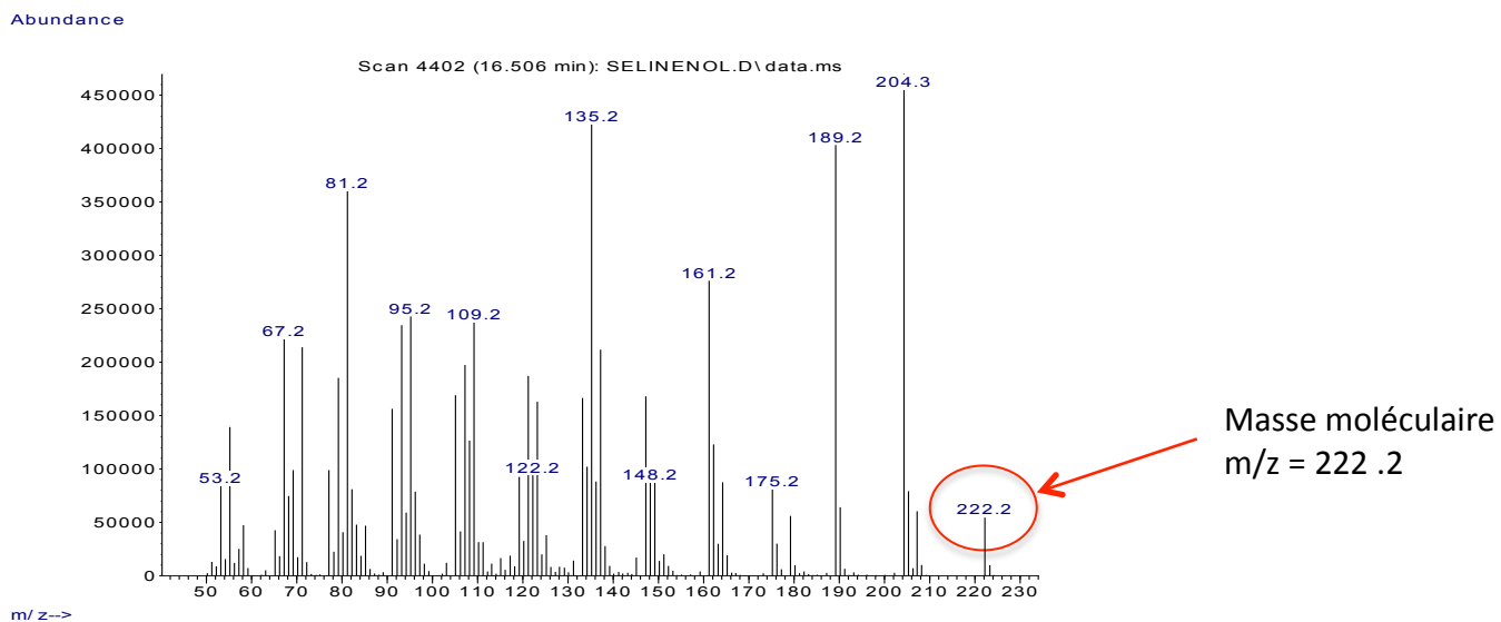
Spectre MS du sélin-11-en-4- \alpha -ol
