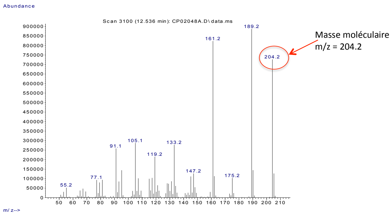
Spectre MS de l'eudesma-4,6-diène
