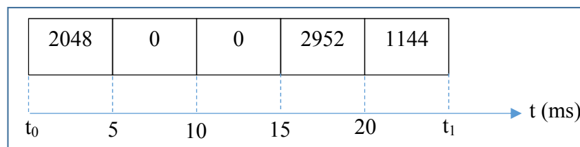
Figure 4.4 Tableau représentant le débit de transmission illustrée par le chronogramme de la figure 4.3
