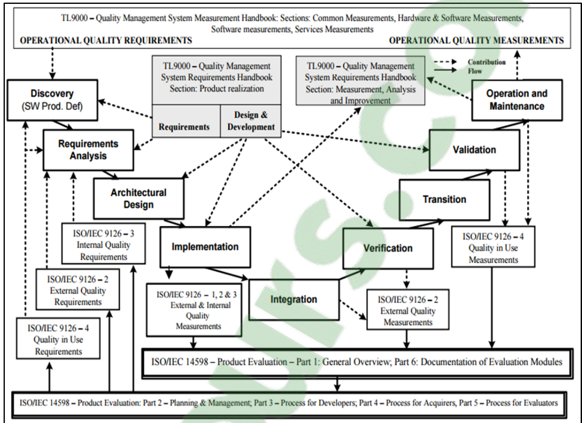
Figure 1.2 Le modèle consolidé de cycle de vie de qualité Suryn-Abran version 0.1
