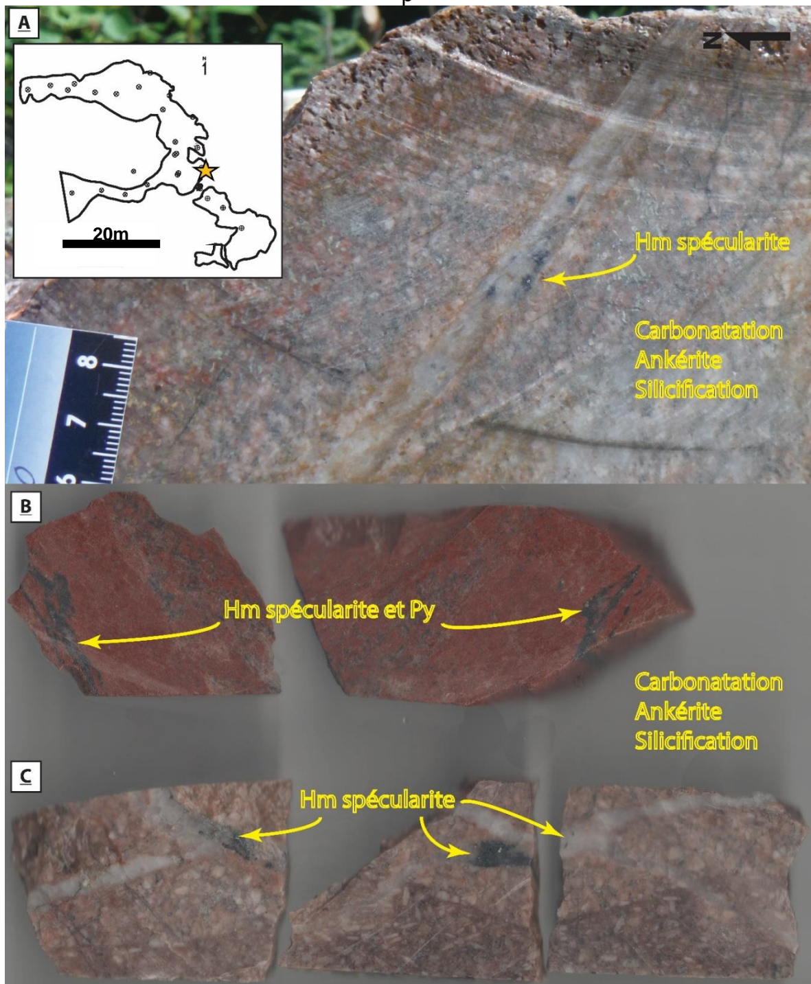
FIGURE 4.6 PRÉSENCE D'HÉMATITE SPÉCULARITE AU SEIN DE VEINES À QUARTZ-CARBONATES: EN AFFLEUREMENT (DÉCAPAGE PRINCIPAL – ÉTOILE POUR EMPLACEMENT (A) ET EN FORAGES (ÉCHANTILON 58_30.2 (B) ET 58_117.5 (C)). LE FORMAT DES CAROTTES DE FORAGE EST BQ (36,5 MM DE DIAMÈTRE).
