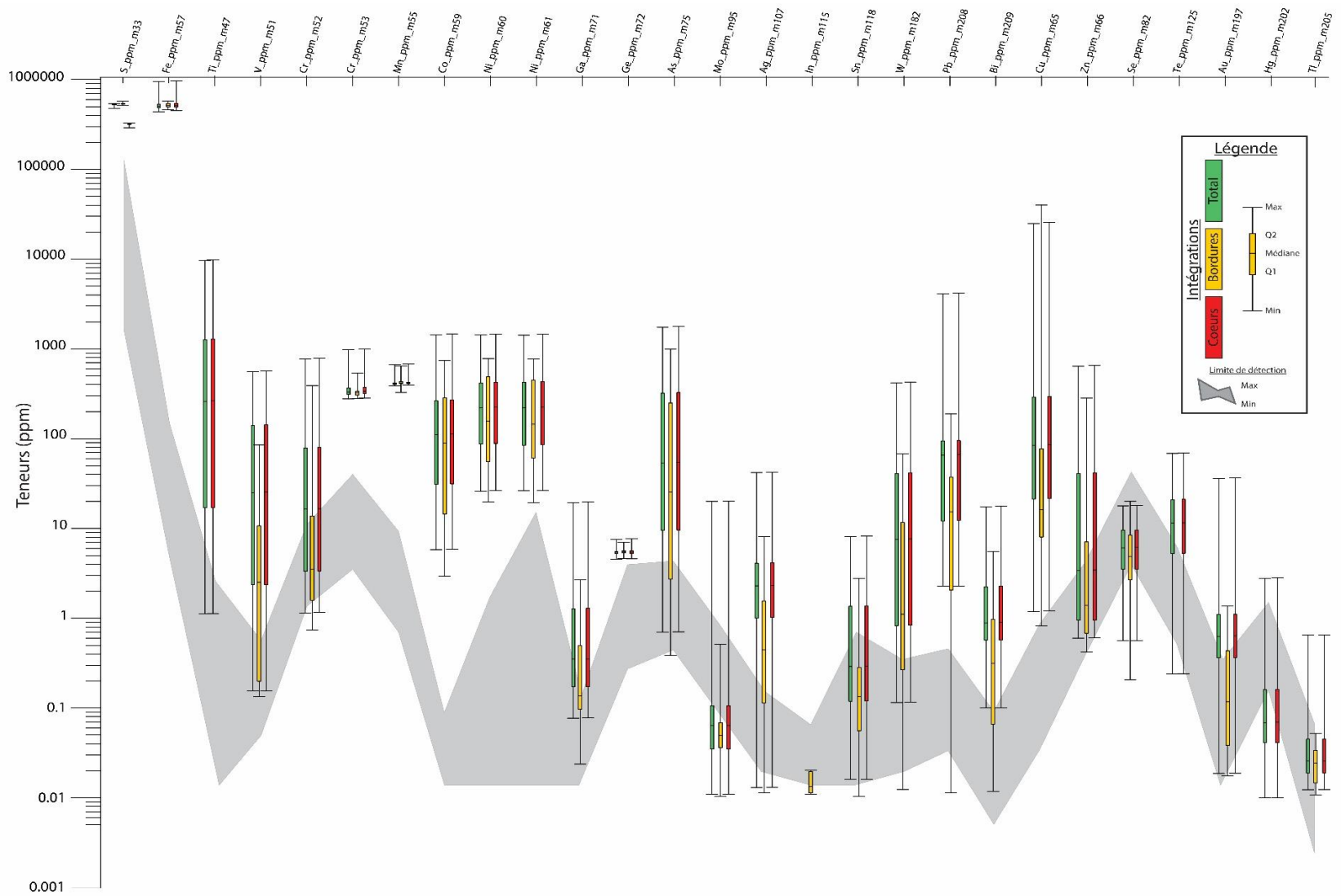
FIGURE 4.19 DIAGRAMMES EN BOÎTES À MOUSTACHES DES VALEURS D'ANALYSE POUR LES GRAINS DE PYRITE (LIGNES TOTALES, COEURS ET BORDURES) AVEC LES LIMITES DE DÉTECTION (MINIMALES ET MAXIMALES).
