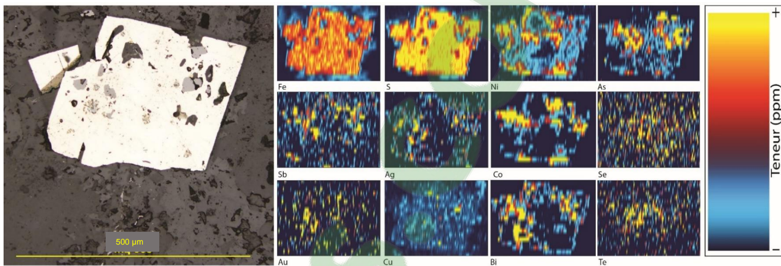
FIGURE 4.8 CARTOGRAPHIE ÉLÉMENTAIRE D'UNE PYRITE DE TYPE 1 ET 2 (BVA-06).
