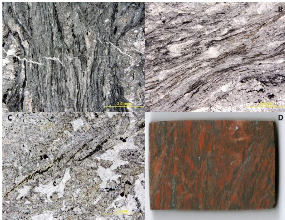
FIGURE 2.18 STRUCTURES DUCTILES - LAME 66_97,5 : CISAILLEMENT OBSERVÉ À PROXIMITÉ DU COULOIR DE DÉFORMATION LAC SHORTT. (A) VEINE DE QUARTZ PLISSÉE ET BOUDINÉE. (B) CISAILLEMENT AVEC FRAGMENTS DE CISAILLEMENTS DANS LES VEINULES DE CHLORITE AU SEIN DES FRAGMENTS MAFIQUES (LAME BVA-23). (D) APERÇU GÉNÉRAL DE LA DÉFORMATION DANS LE BLOC DE LA LAME MINCE 66_97,5.
