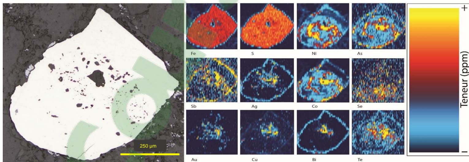
FIGURE 4.9 CARTOGRAPHIE ÉLÉMENTAIRE D'UNE PYRITE DE TYPE 1 ET 2 (62_448)
