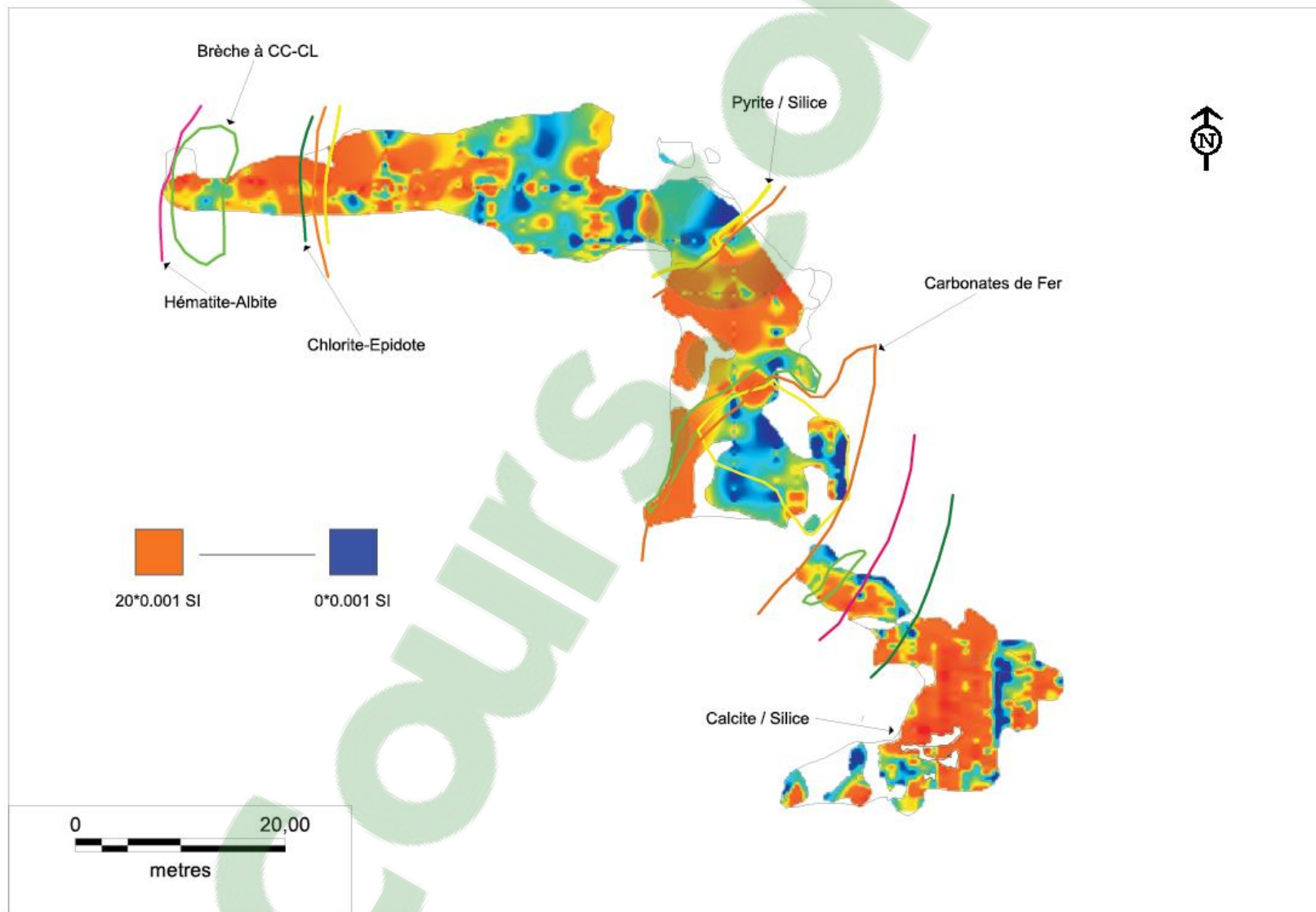
FIGURE 3.14 CARTOGRAPHIE DE LA SUSCEPTIBILITÉ MAGNÉTIQUE AVEC ALTÉRATIONS HYDROTHERMALES DU DÉCAPAGE PRINCIPAL
