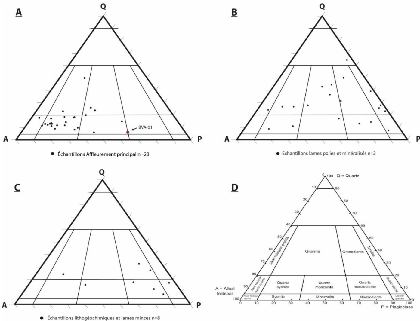
FIGURE 2.10 CLASSIFICATION MINÉRALOGIQUE DES ÉCHANTILLONS (STRECKEISEN, 1976) A) ÉCHANTILLONS DU DÉCAPAGE PRINCIPAL; B) ÉCHANTILLONS MINÉRALISÉS EN OR; C) ÉCHANTILLONS « FRAIS » UTILISÉS POUR LITHOGÉOCHIMIE ET D) CHAMPS LITHOLOGIQUES DÉFINIS PAR STRECKEISEN (1967)
