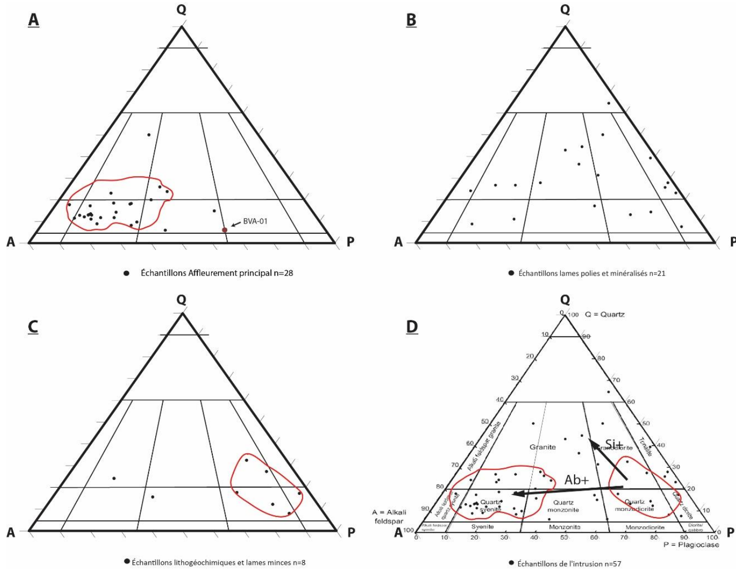
FIGURE 6.1 INTERPRÉTATION DE LA MIGRATION DES PÔLES MINÉRALOGIQUES PRODUITS PAR L'ALTÉRATION HYDROTHERMALE.
