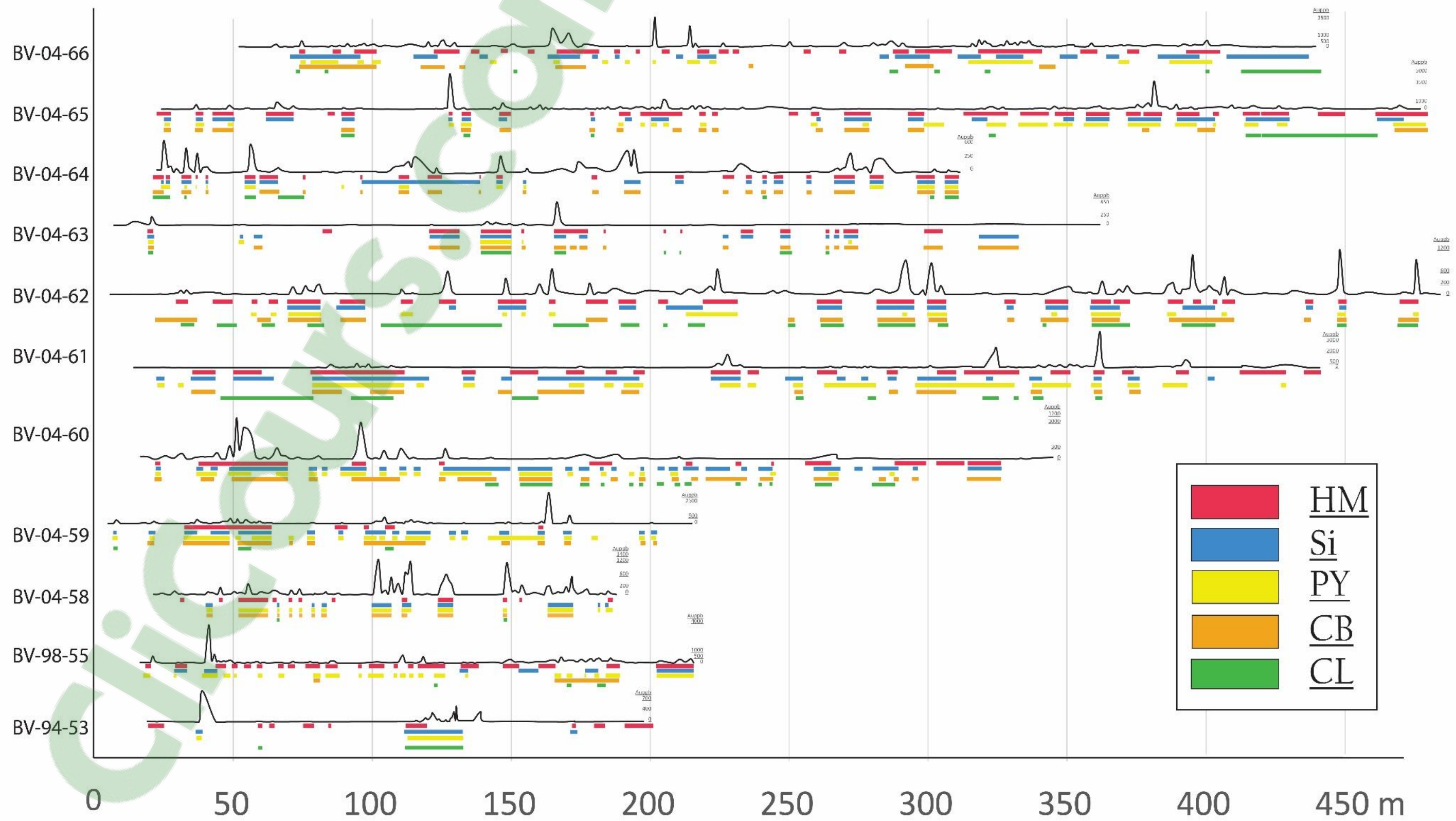
FIGURE 34 INTERVALLES D'ALTÉRATION HYDROTHERMALE EN FORAGE AVEC ANALYSES AURIFÈRES (NOR). LES ÉCARTS POUR LES ANALYSES AURIFÈRES SONT VARIABLES À CHAQUE TROU DE FORAGE
