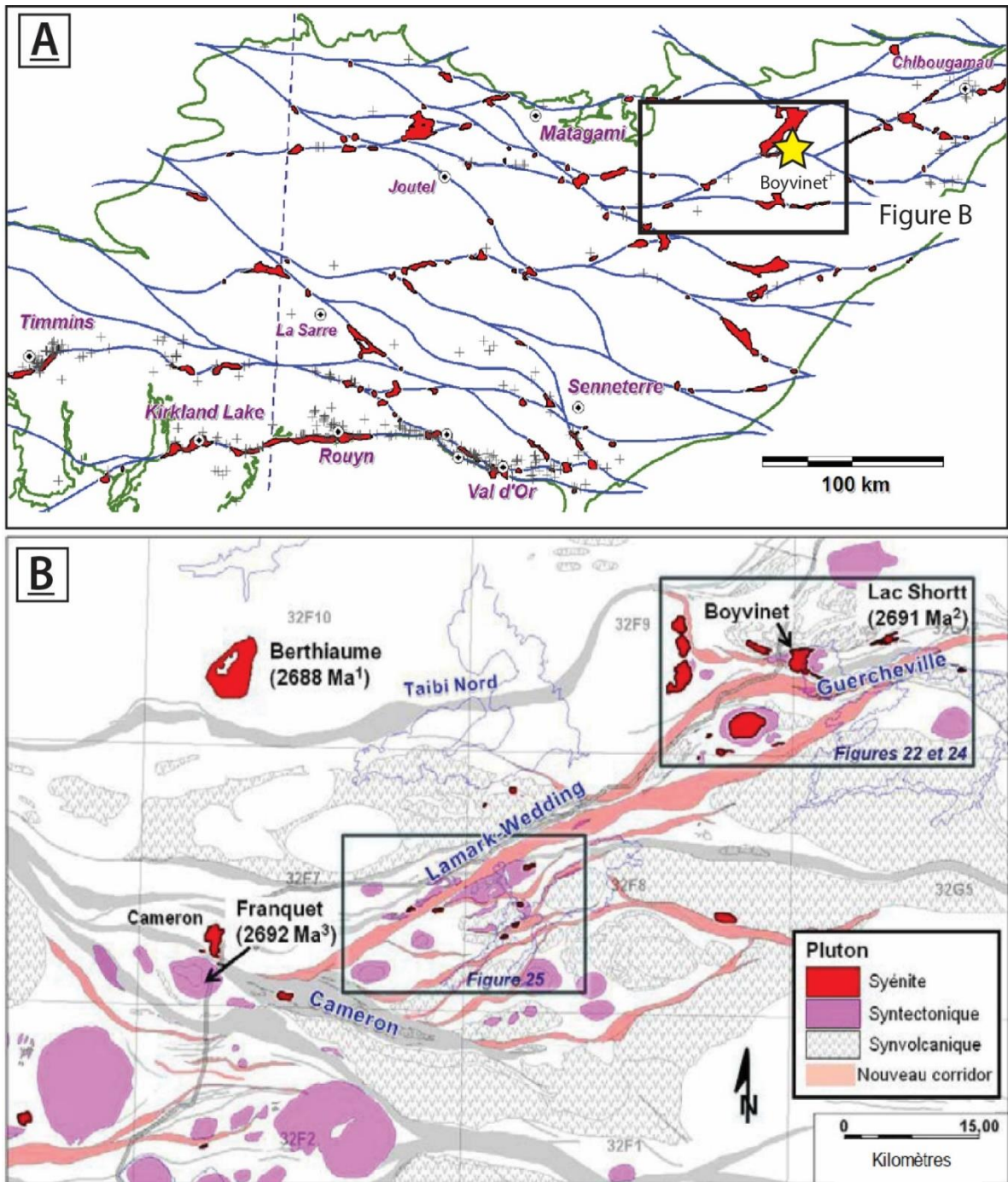
FIGURE 6.7 (A) ZONES CIBLÉES POUR LES MINÉRALISATIONS DE TYPE OROGÉNIQUE PAR FAURE ET AL. (2008). EN ROUGE LES ZONES CIBLÉES, LES CROIX ÉTANT DES GÎTES AURIFÈRES CONNUS. (B) TYPOLOGIES DES INTRUSIONS DANS LE SECTEUR DE LABEL-SUR-QUÉVILLON / LAC SHORTT DÉFINIS PAR FAURE (2011). NOTEZ LA PRÉSENCE DE NOMBREUX PLUTONS SYNVOLCANIQUES ET SYÉNITIQUES. LE STOCK DE BOYVINET Y EST PRÉSENTÉ COMME UNE SYÉNITE
