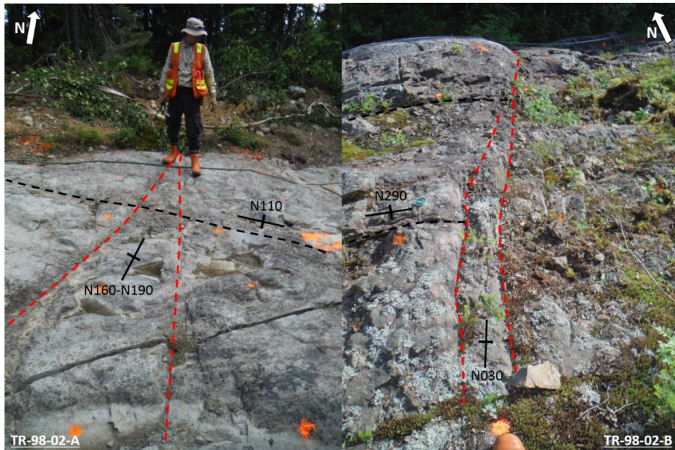
FIGURE 2.14 STRUCTURES OBSERVÉES DANS LA PARTIE EST DE L'INTRUSION (DÉCAPAGES TR-98-02-A & B). STRUCTURES N-S ET E-O; BOTTE À DROITE POUR ÉCHELLE.
