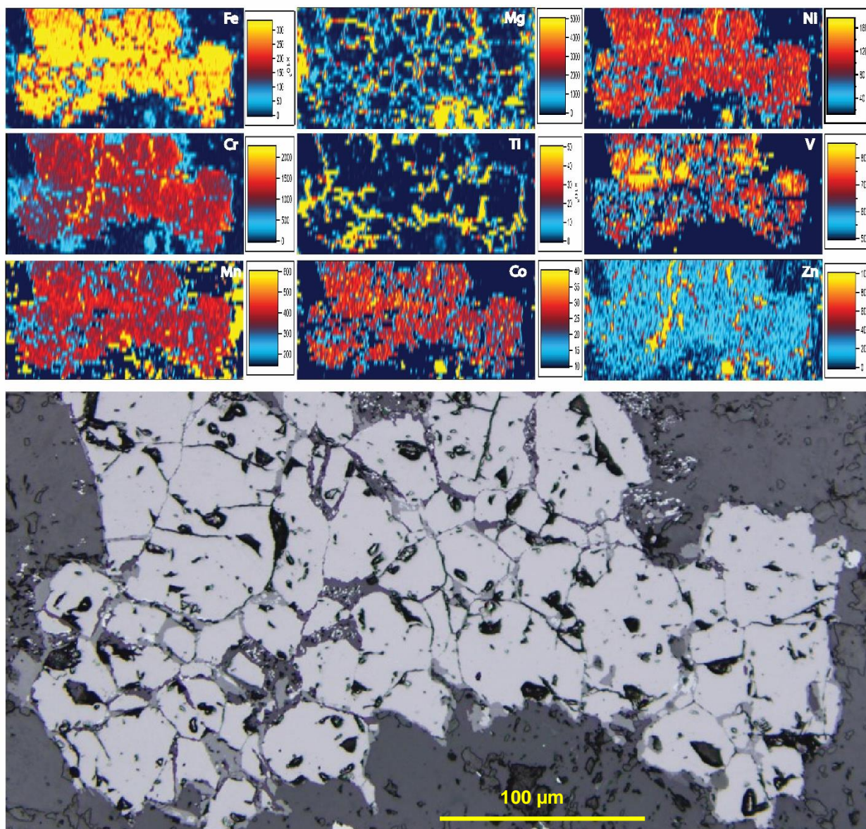
FIGURE 4.13 CARTOGRAPHIE ÉLÉMENTAIRE D'UN GRAIN D'OXYDE (ÉCH. BVA-26) VALEURS EN PPM.
