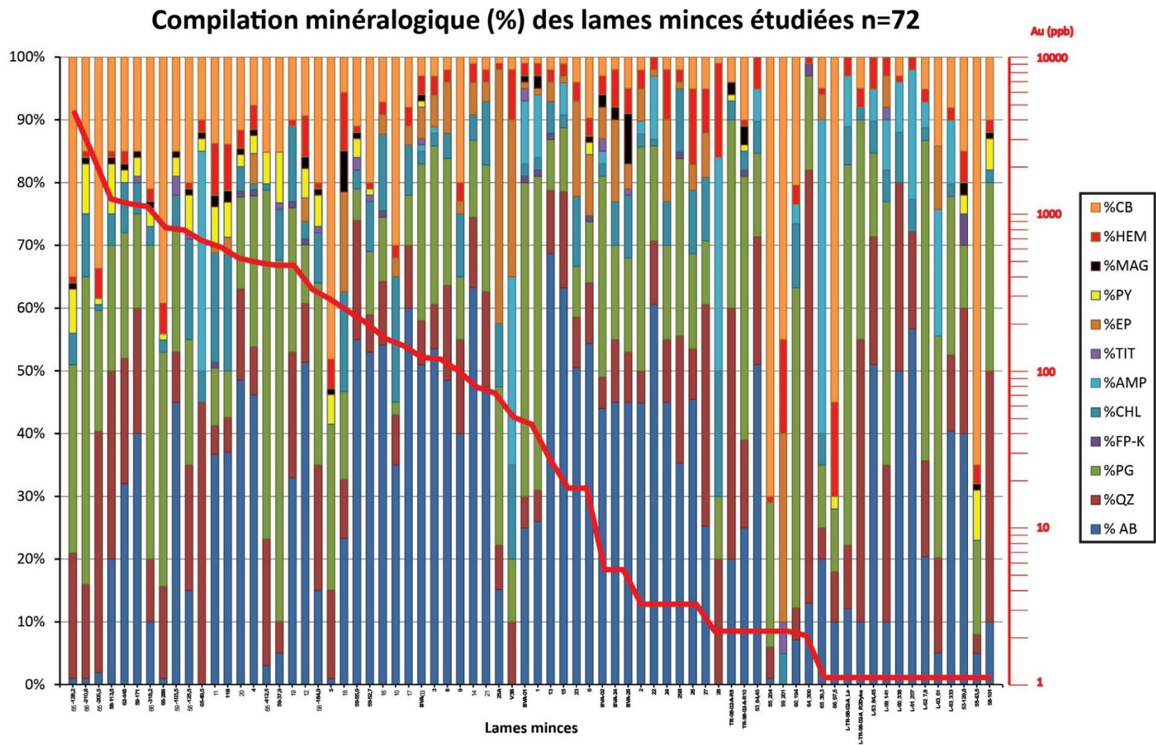
FIGURE 2.2 DIAGRAMME À BARRES DE LA COMPILATION DES POURCENTAGES MINÉRALOGIQUES DES LAMES MINCES ÉTUDIÉES (N=72) AVEC ANALYSES EN AU (PPB) SUPERPOSÉES.
