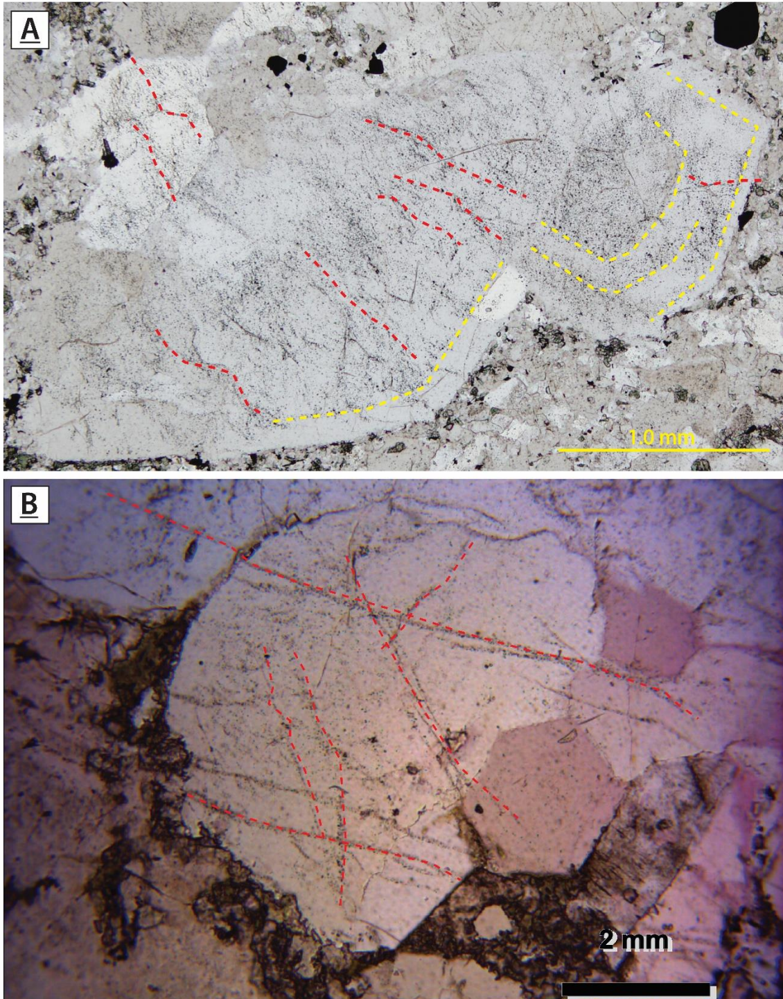
FIGURE 5.4 TYPOLOGIE DES INCLUSIONS FLUIDES SELON ROEDDER (1979) : (A) PRIMAIRES EN JAUNE ET PSEUDOSECONDAIRES/SECONDAIRES EN ROUGE (ÉCHANTILLON 59_55.9). (B) INCLUSIONS SECONDAIRES (SÉCANTES À PLUSIEURS GRAINS) ET PSEUDOSECONDAIRES (DANS UN SEUL GRAIN) EN ROUGE (ÉCHANTILLON BVA20).
