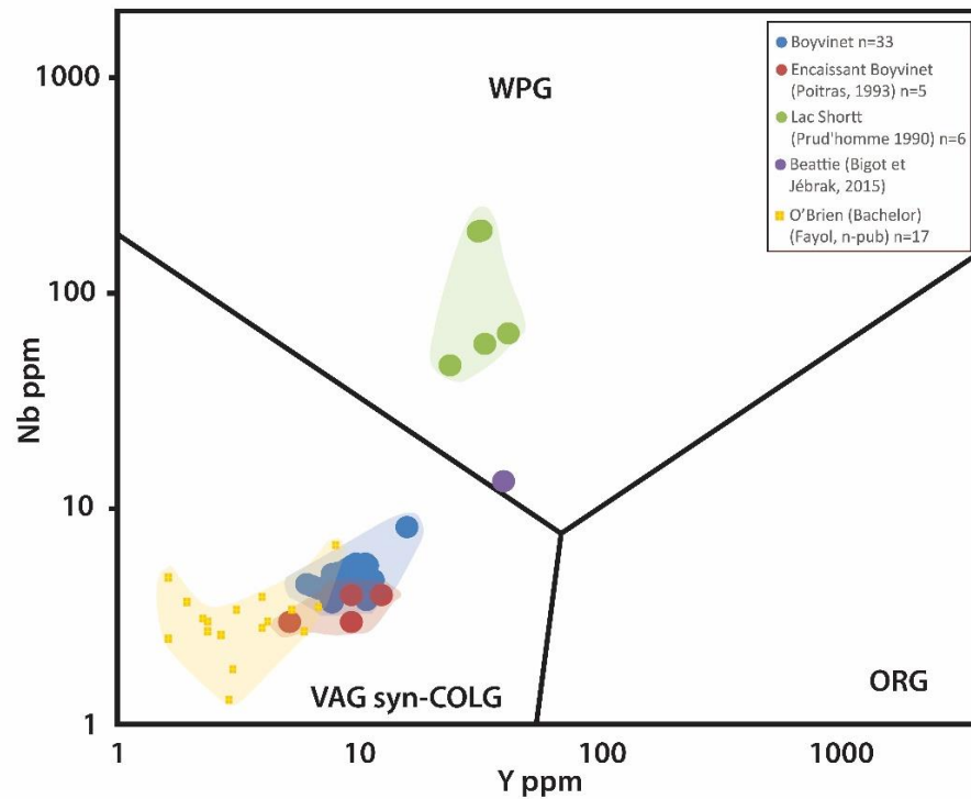
FIGURE 2.13 DIAGRAMME NB VS Y POUR LE CONTEXTE TECTONIQUE DE MISE EN PLACE POUR L'INTRUSION ET L'ENCAISSANT (POITRAS, 1993); MODIFIÉ DE PEARCE (1984)
