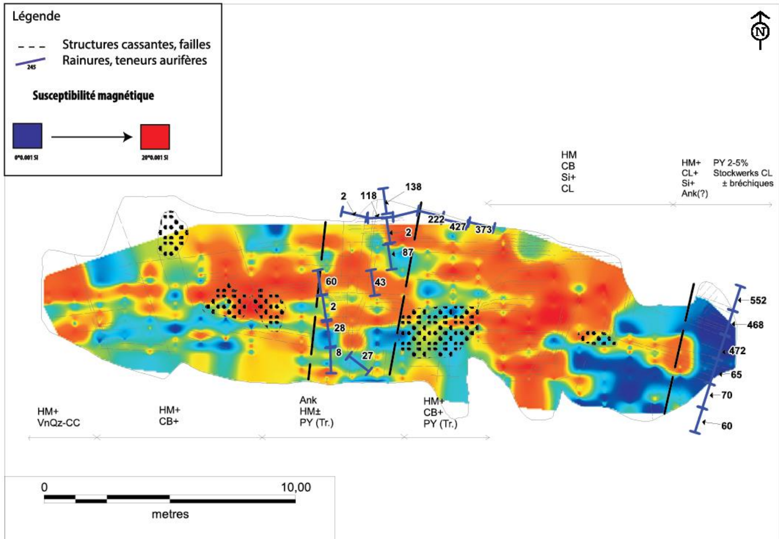
FIGURE 3.13 CARTOGRAPHIE DE LA SUSCEPTIBILITÉ MAGNÉTIQUE AVEC STRUCTURES, ALTÉRATIONS HYDROTHERMALES, RAINURES ET TENEURS AURIFÈRES (PPB) DE L'AFFLEUREMENT TR-98-02-B
