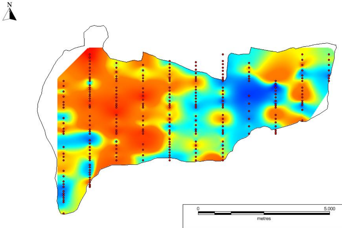
FIGURE 3.9 EXEMPLE DE TRAITEMENT DES DONNÉES DE SUSCEPTIBILITÉ MAGNÉTIQUE SUR L'AFFLEUREMENT TR-98-02-A (PARTIE OUEST)
