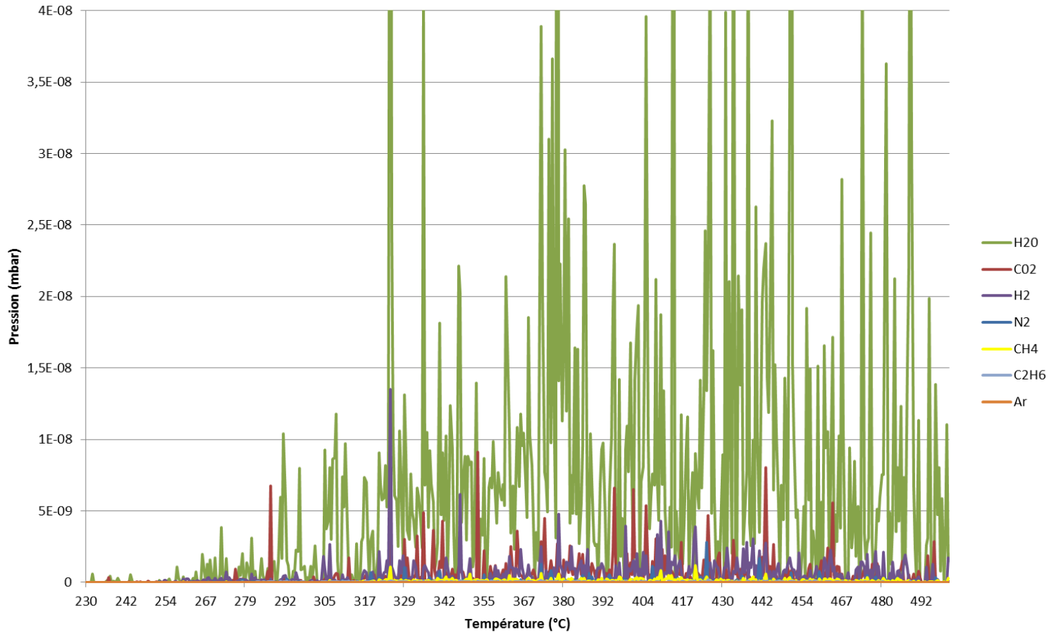
FIGURE 5.6 GRAPHIQUE DES DONNÉES D'ANALYSE PAR SPECTROMÉTRIE DE MASSES À SONDE SOLIDE (PRESSION (MBAR) EN FONCTION DE LA TEMPÉRATURE) AVEC LA RÉDUCTION DU BRUIT DE FOND. UNE INCRÉMENTATION DE 6 DEGRÉS PAR MINUTE EST UTILISÉE (SELON GABOURY ET AL., 2008). CHAQUE PIC OBSERVÉ ÉQUIVAUT À LA DÉCRÉPITATION D'INCLUSIONS FLUIDES, ET LA SOMMATION DE TOUS CES PICS CORRESPOND À LA PRESSION PARTIELLE DES GAZ DANS L'ANALYSE.
