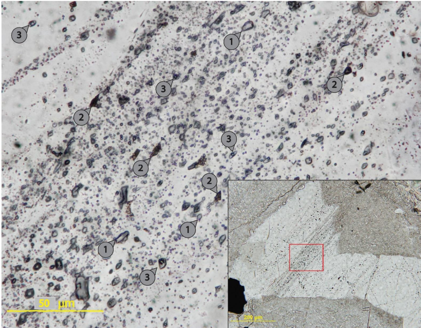
FIGURE 5.5 EXEMPLE COMMUN DES TYPES D'INCLUSIONS FLUIDES RENCONTRÉES DANS LES GRAINS DE QUARTZ AU SEIN DU STOCK DE BOYVINET : IF1 (DOMINANCE LIQUIDE); IF2 (DOMINANCE GAZEUSE) ET IF3 (LIQUIDE+GAZ). ÉCHANTILLON 59_171.
