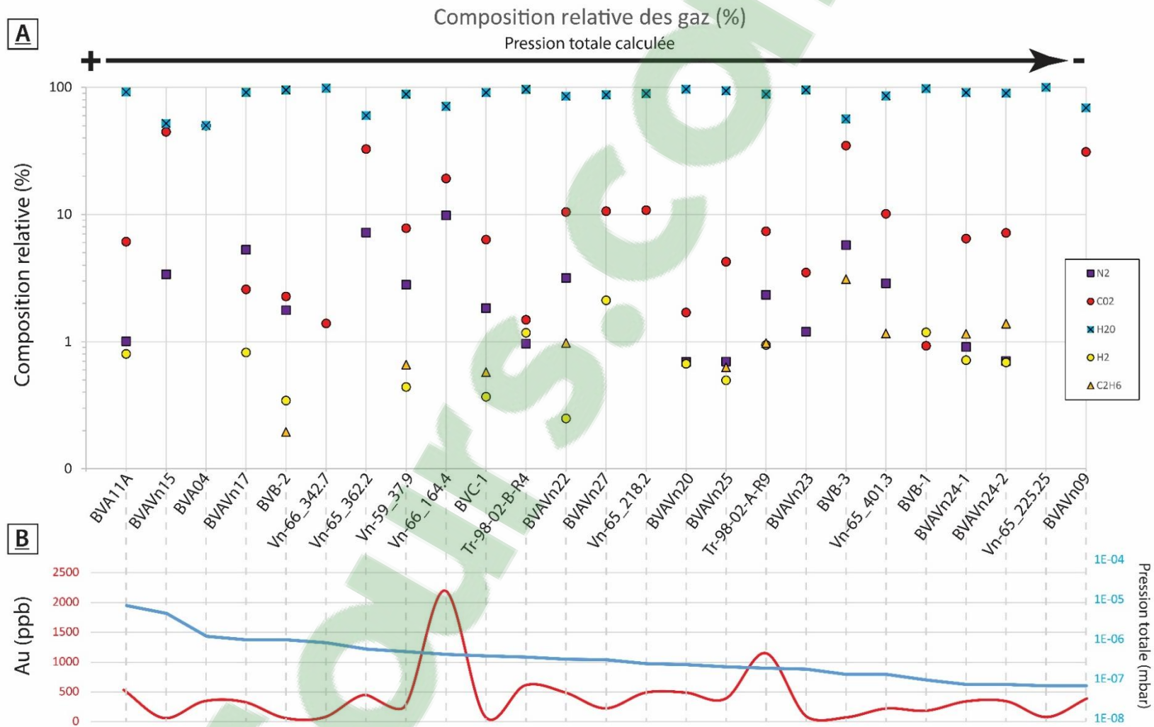
FIGURE 5.7 (A) GRAPHIQUE DE LA COMPOSITION EN GAZ DES 24 ÉCHANTILLONS PLACÉS EN ORDRE DÉCROISSANT DE PRESSION TOTALE (MBAR) DES GAZ CALCULÉE. (B) TENEURS AURIFÈRES (AU PPB) RELIÉES À CHAQUE ÉCHANTILLON, AVEC LA PRESSION TOTALE (MBAR).
