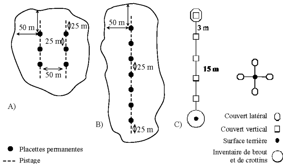
Figure 2. Design expérimental établi dans 12 peuplements témoins et dans 20 éclaircies commerciales en Abitibi, Québec, 2006-2007. A) Design dans les sites de forme carrée, B) Design dans les sites de forme rectangulaire, C) Plan d'inventaire à chacune des placettes.
