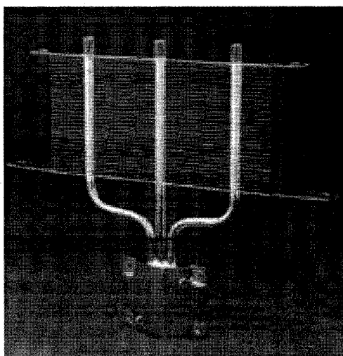
Figure 2 Caloducs avec ailettes Thermo-Sink (Source : Thermaco)
