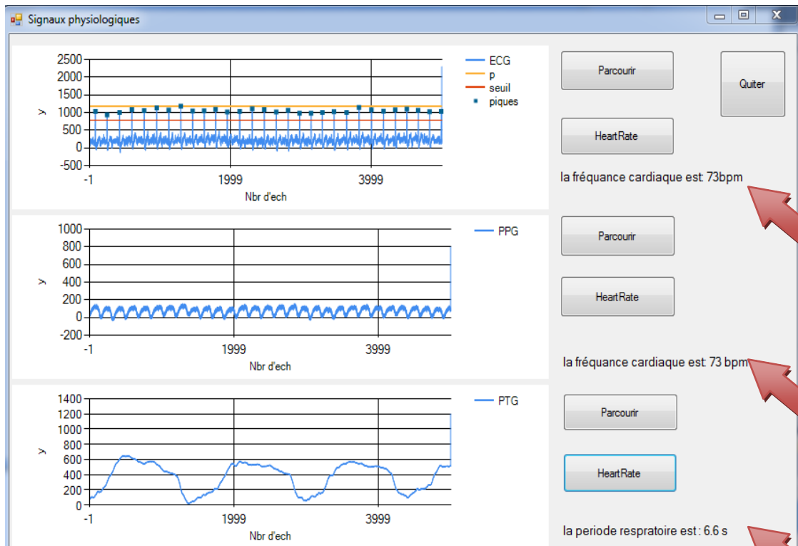
Figure IV.19: Calcul des différents paramètres physiologiques.
