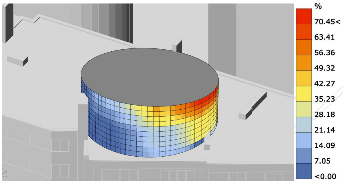
Fig. 45 : Accès visuel au paysage vue (Vue SE)
