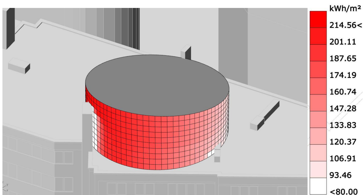
Fig. 44 : Apports énergétiques surfaciques solaires en KWh/m 2 lorsque la température est supérieure à 18°C
