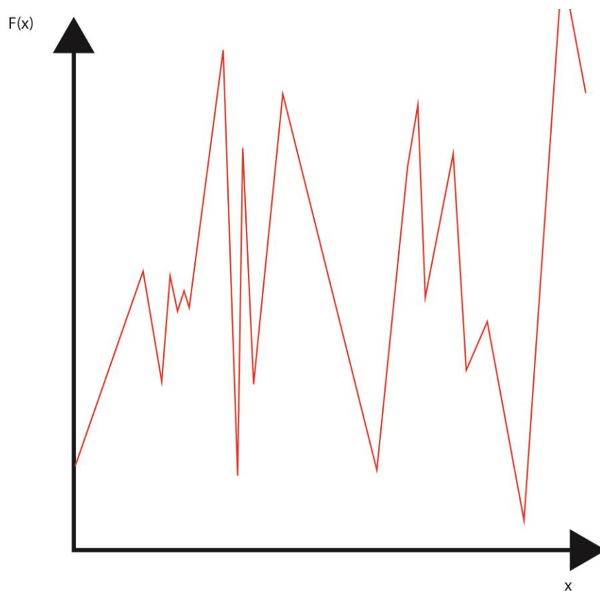
Fig. 29 : Exemple de fonction discontinue
