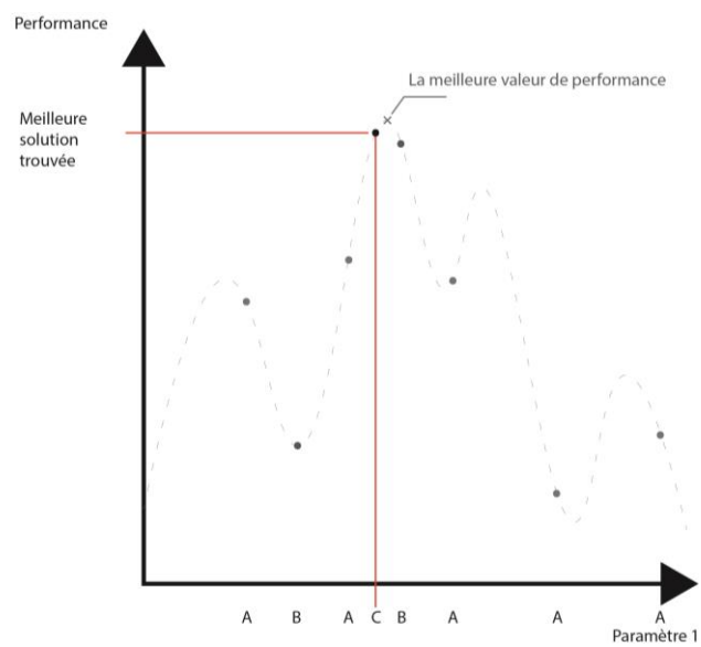
Fig. 17 : Exemple de recherche d'un optimum par recherche directe.
