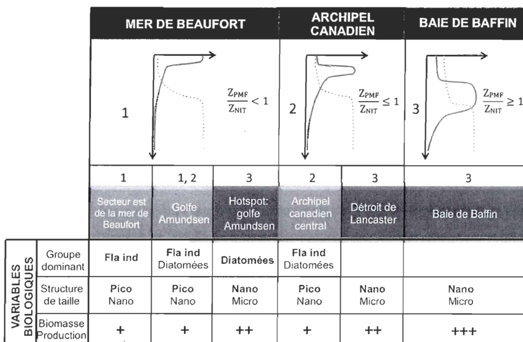
Fig. 1: Modèle conceptuel des profils verticaux typiques des concentrations de la chlorophylle a et du nitrate présentés selon les différentes régions biogéographiques du Haut-Arctique canadien avec leurs caractéristiques biologiques respectives. Fla ind = flagellés indéterminés, Pico = picophytoplancton, Nano = nanophytoplancton, Micro = microphytoplancton; case gris foncée = région eutrophe, case gris claire = région oligotrophe, +++ > ++ > + = Intensité de la production et biomasse phytoplanctonique.
