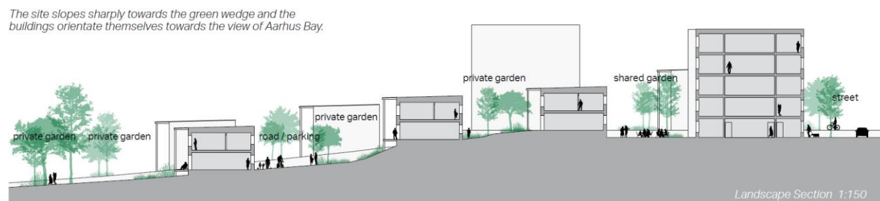
Figure 57 : Coupe du complexe de logements (Source : Circle House)
