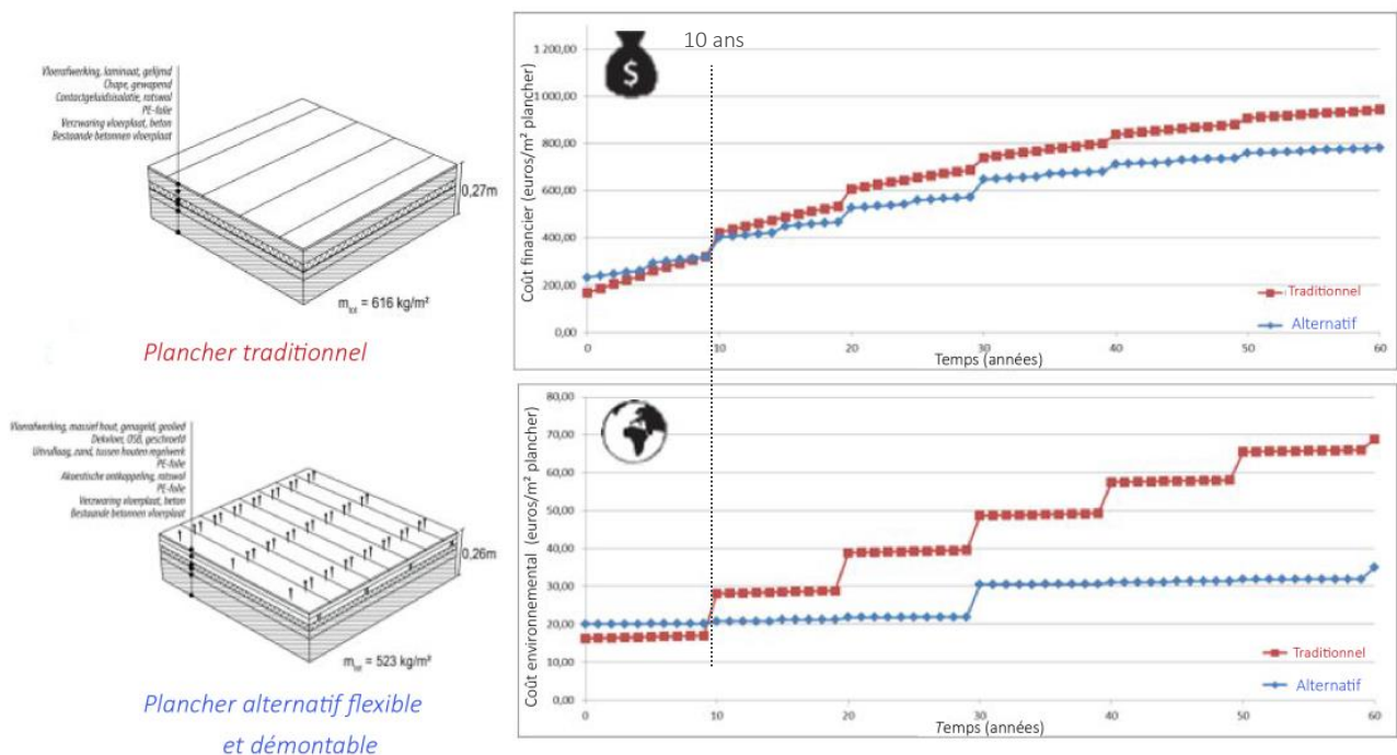
Figure 10 : Comparaison du coût financier et environnemental d'un plancher traditionnel et un plancher alternatif flexible et démontable (Source : traduction de l'étude d'Ovam)
