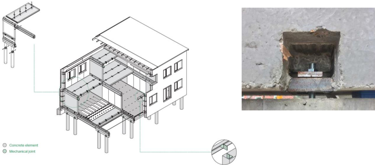
Figure 59 : Système constructif (Source : The Circle House)
