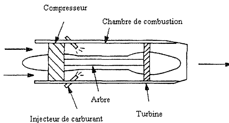
Figure 11 Schéma d'un turboréacteur [3]
