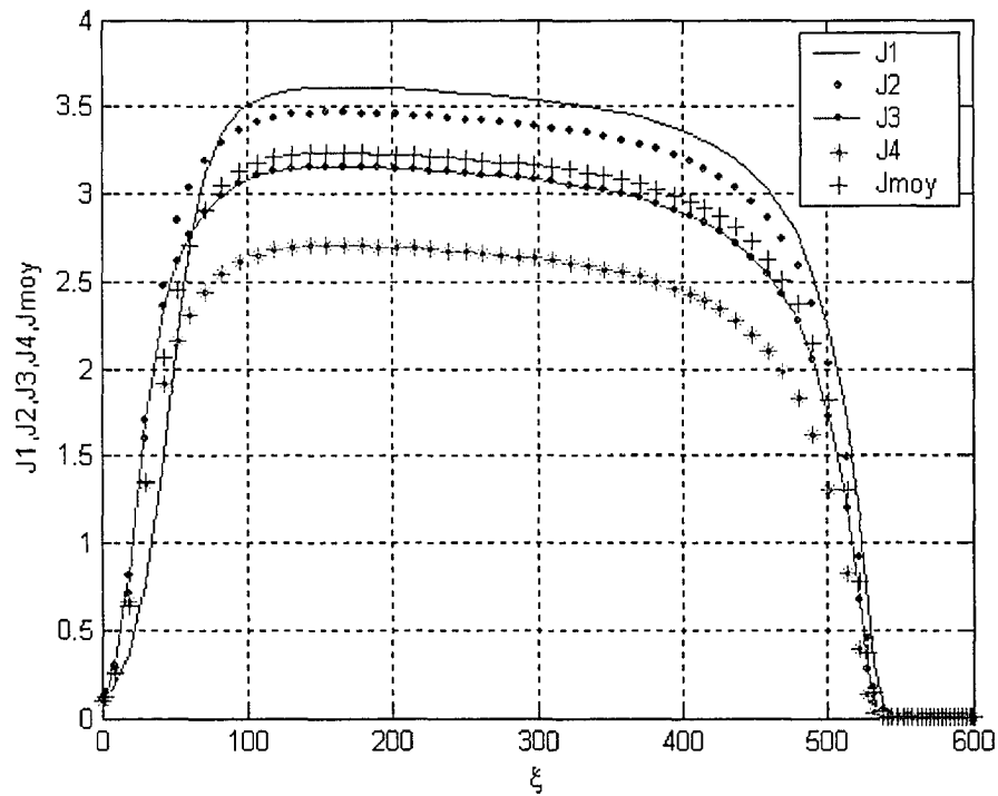
Figure 40 Amplitudes du décrochage tournant pour les différents modes
