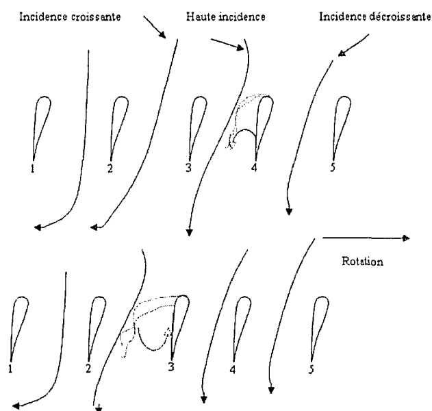
Figure 17 Illustration du phénomène de décrochage tournant
