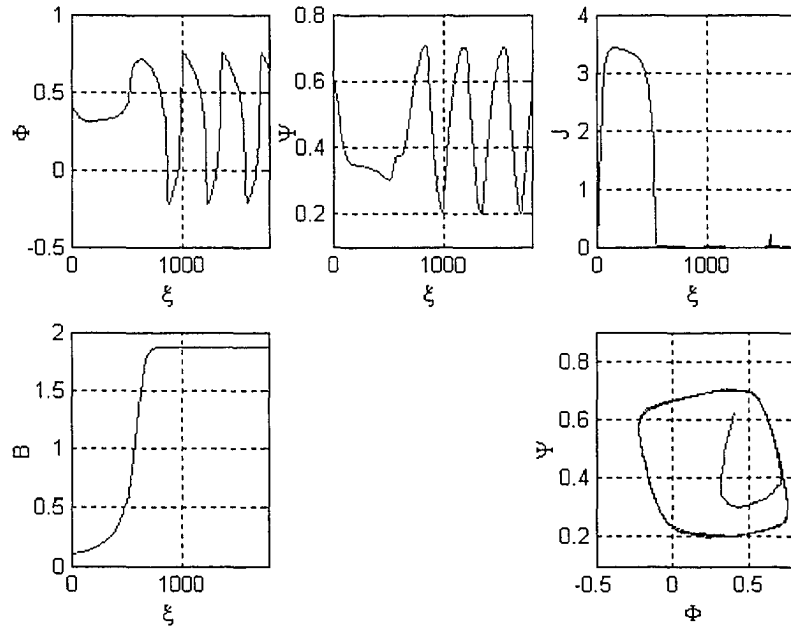
Figure 34 Simulation du modèle de G-E à trois modes pour \gamma = 0.5
