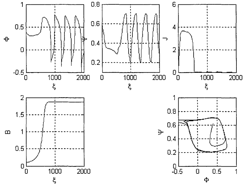
Figure 32 Simulation du modèle de G-E à un seul mode pour \gamma = 0.5
