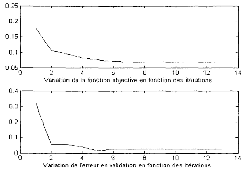
a) Avec le gradient total (Équation 3.6)
