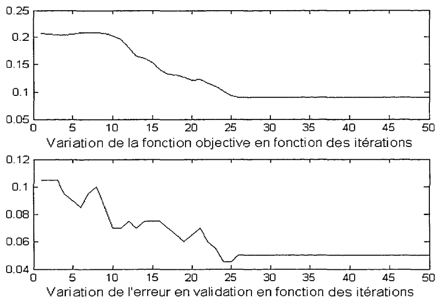
(a) Avec le gradient total (Équation 3.6)
