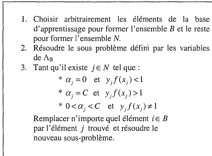
Figure 8 Algorithme de décomposition pour l'apprentissage des SVMs (extraite de [26])
