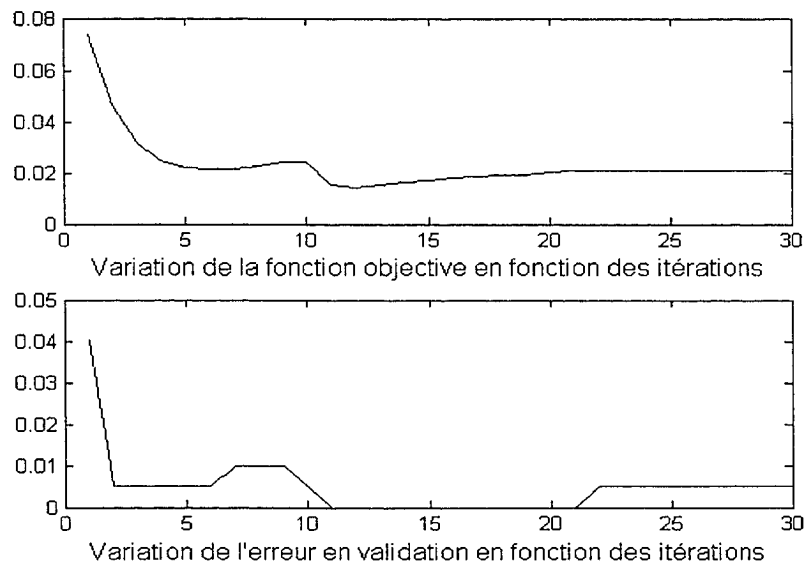
(b) Avec le gradient approché (Équation 3.8)
