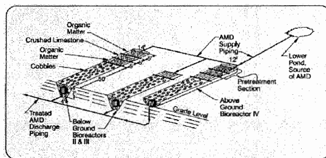
Figure 3 : Vue isométrique des 3 bioréacteurs (MSE Technology Application Inc., 2002).
