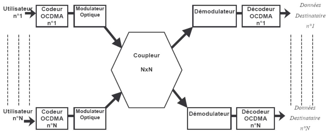
Figure I.7 : réseau OCDMA
