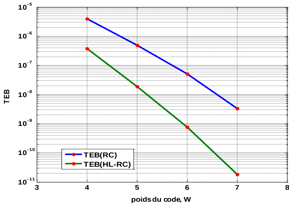
Figure III. 9: La probabilité d'erreur P_{\text{ERC}} et P_{\text{eHL-RC}} , en fonction du poids de code pour un code OOC (361, W, 1) et N=8
