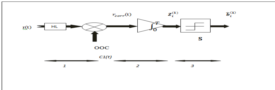
Figure II. 9 : Récepteur Conventionnel avec limiteur de l'utilisateur 1
