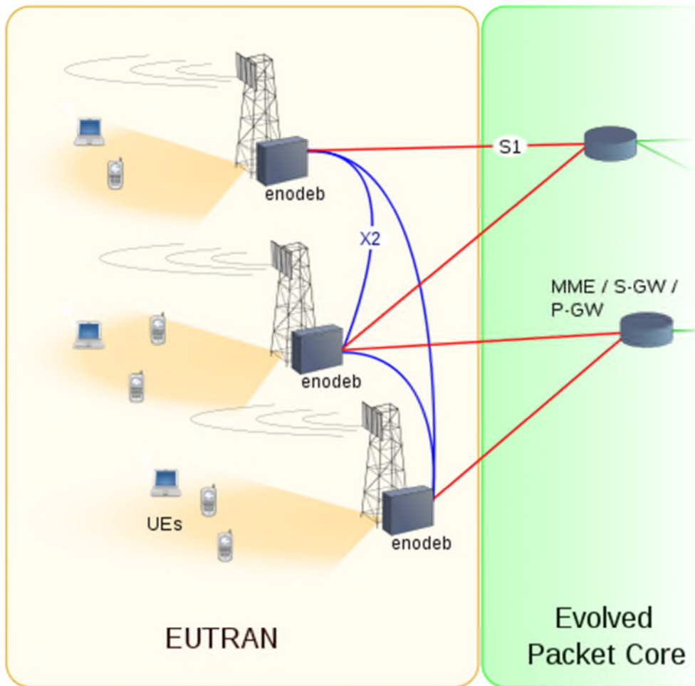
Figure 1.14 : architecture d'un reseau LTE(4G)
