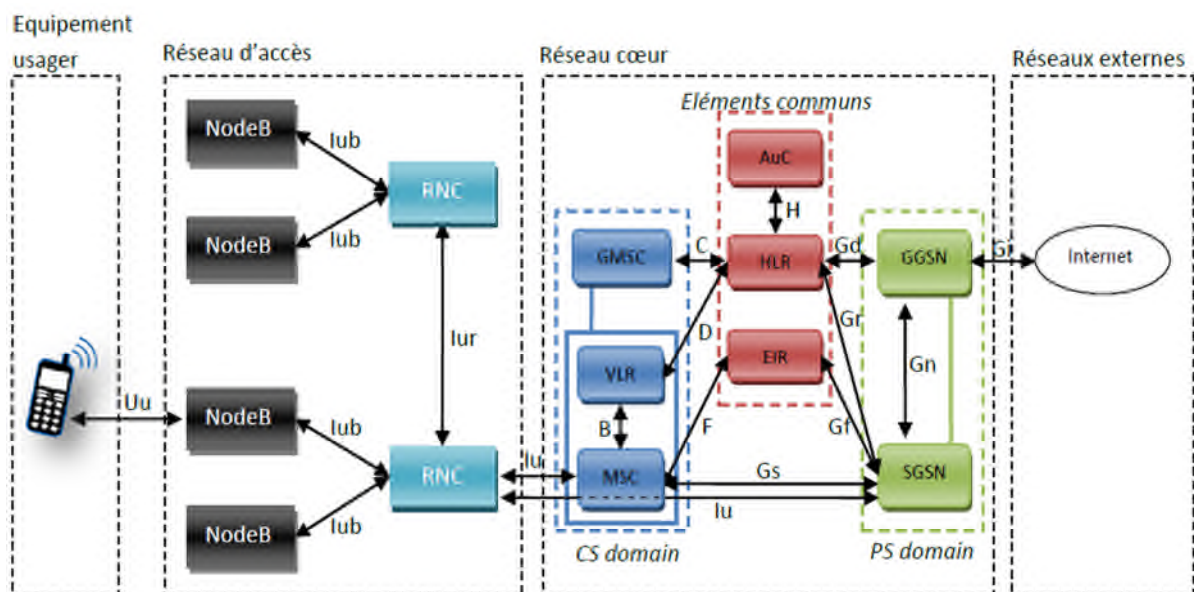
Figure 1.11 : architecture d'un reseau UMTS(3G)
