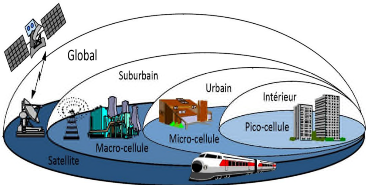
Figure 1.12 : Hiérarchie des cellules de l'UMTS
