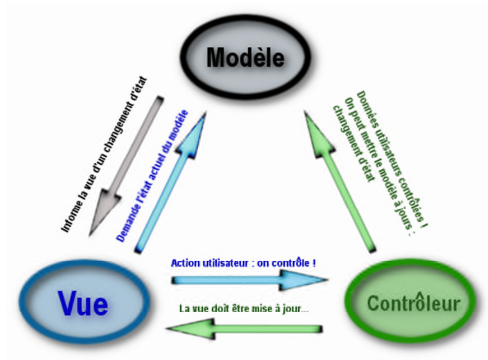
Figure 2.5 : modèle MVC
