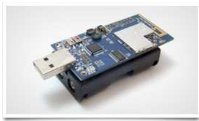
Figure IV.5 Spécifications de capteur MTM-CM5000MSP .
