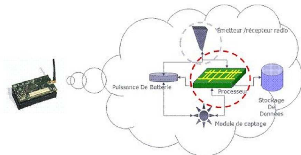
Figure I.2 Anatomie d'un nœud capteur. [3]
