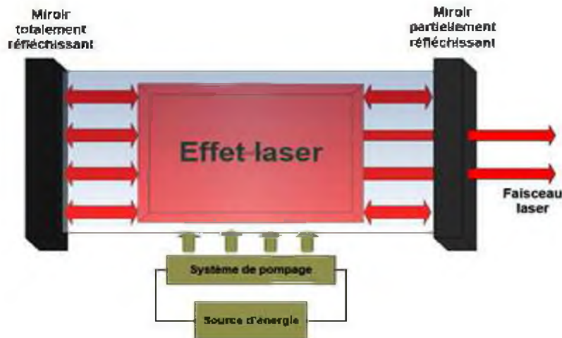
Figure 1.3 Principe de fonctionnement d'un laser
