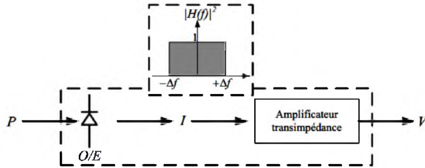
Figure 3.5 Schéma de principe de la conversion d'une puissance optique P vers une tension V à l'aide d'un photodétecteur intégrant un amplificateur transimpédance
