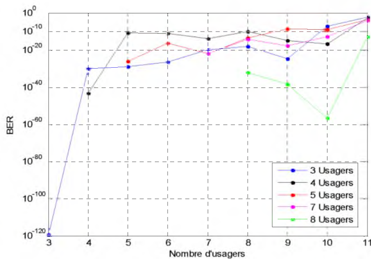
Figure 4.40 BER en fonction du nombre d'utilisateur
