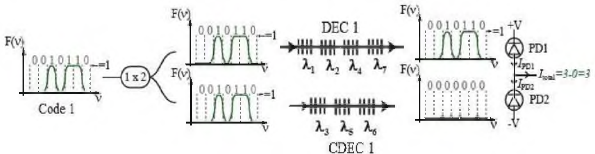
Figure 3.2 Fonctionnement du système de décodage de l'utilisateur 1 pour un signal émis avec le code 1
