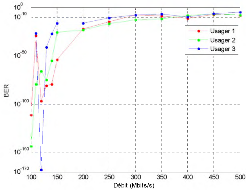
Figure 4.25 BER en fonction du débit binaire pour 3 utilisateurs
