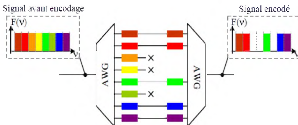
Figure 3.7 Encodage SAC-OCDMA à base d'AWGs
