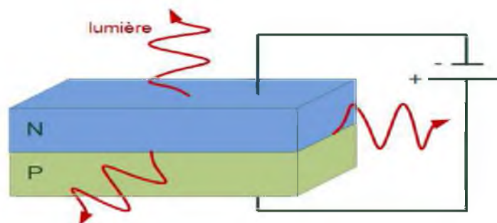
Figure 1.2 Schéma simplifié d'une diode électroluminescente
