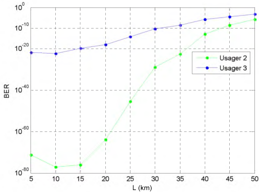
Figure 4.15 BER en fonction de L (1 éteint, 2 et 3 allumés)
