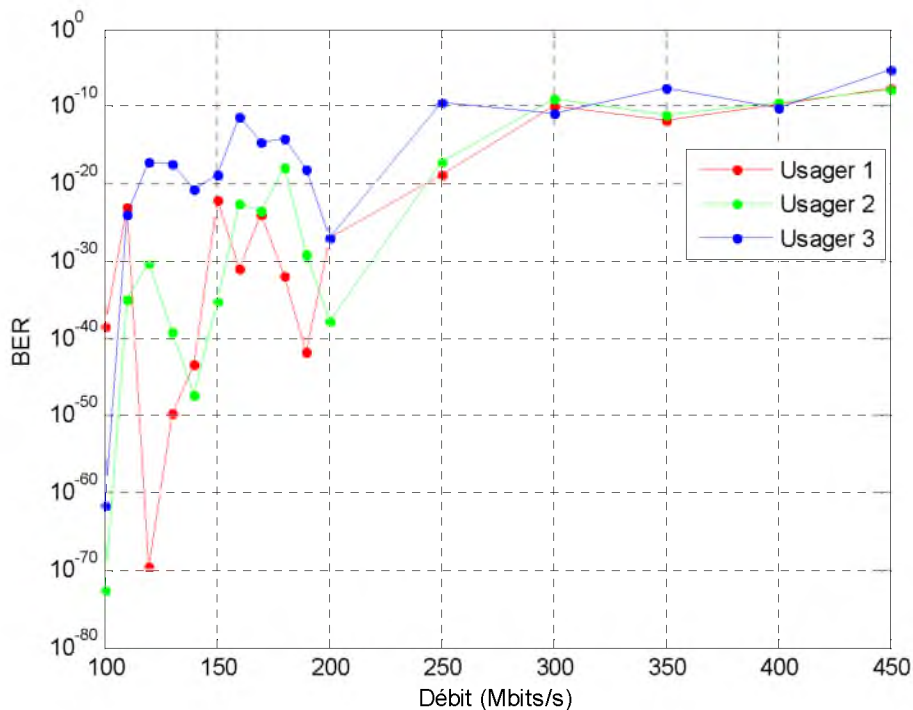
Figure 4.34 BER en fonction du débit binaire
