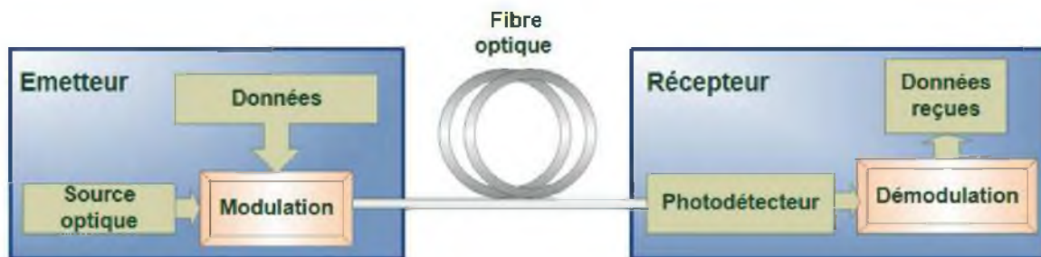
Figure 1.1 Synoptique générale d'un système de communication par fibre optique
