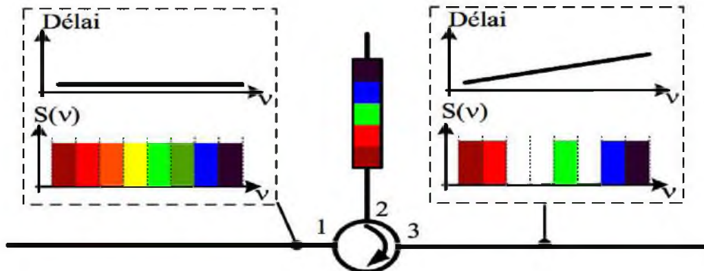
Figure 3.10 Cascade de deux réseaux pour encodage SAC-CDMA
