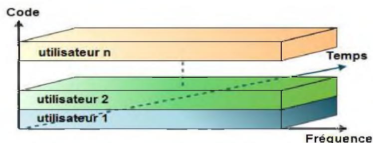
Figure 2.9 Représentation temps/fréquence du CDMA en fonction des codes utilisateurs
