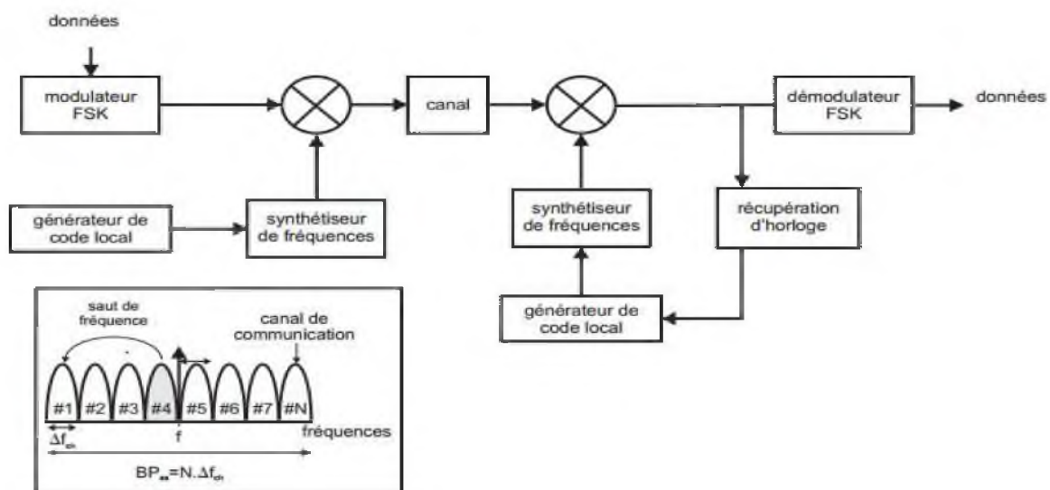
Figure 2.8 Encodeur et décodeur FH-SS, spectre du signal étalé
