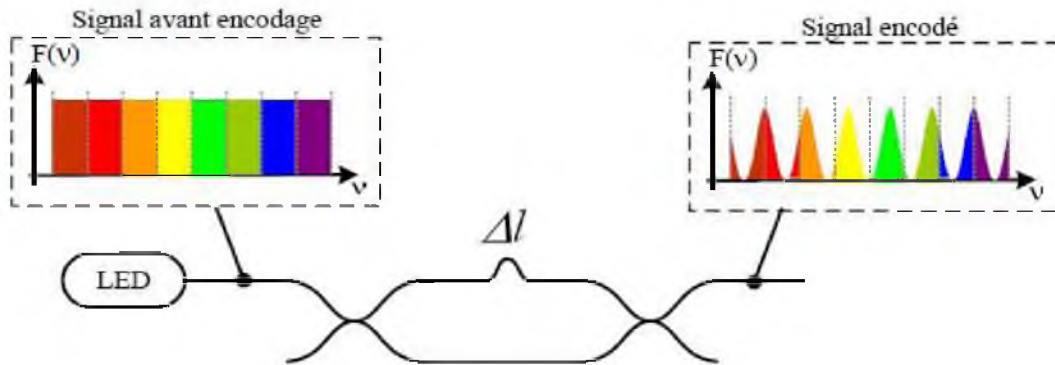
Figure 3.8 Encodage SAC-OCDMA utilisant un interféromètre de Mach-Zehnder
