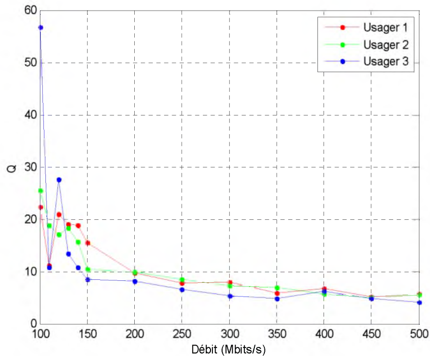
Figure 4.26 Q en fonction du débit binaire pour 3 utilisateurs
