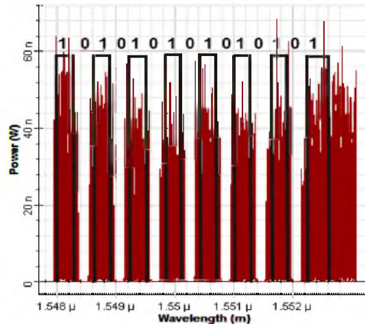
Figure 4.36 Code avec des bits « 1 » isolés
