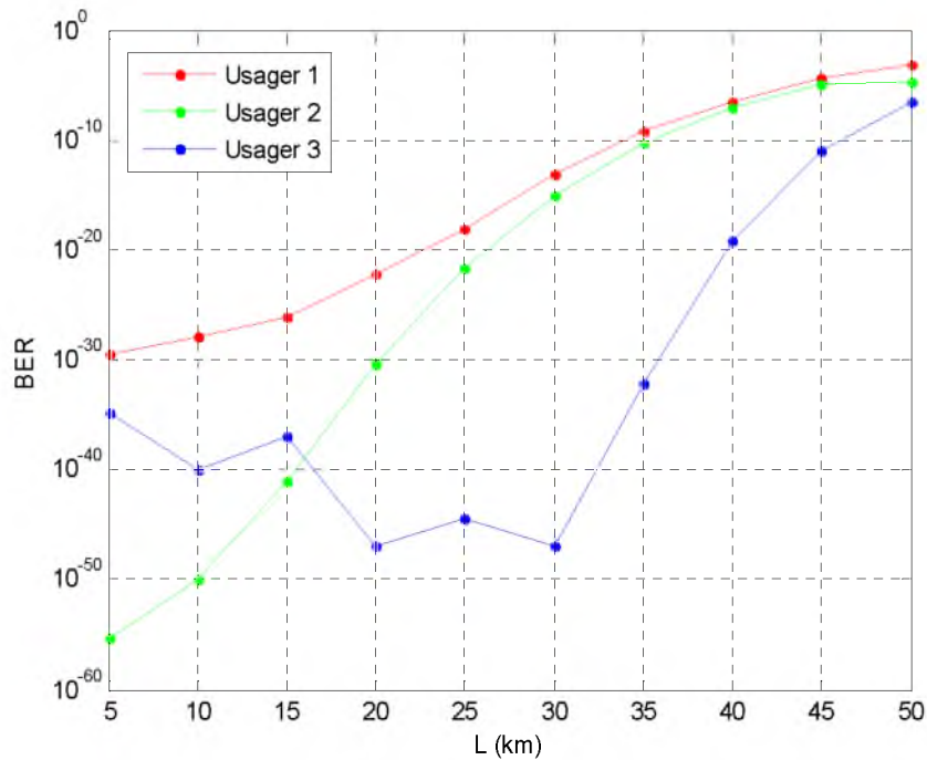
Figure 4.29 BER en fonction de la longueur de la fibre optique
