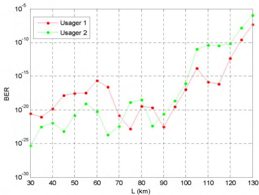
Figure 4.20 BER en fonction de la longueur de la fibre optique (3 éteint, 1 et 2 allumés)
