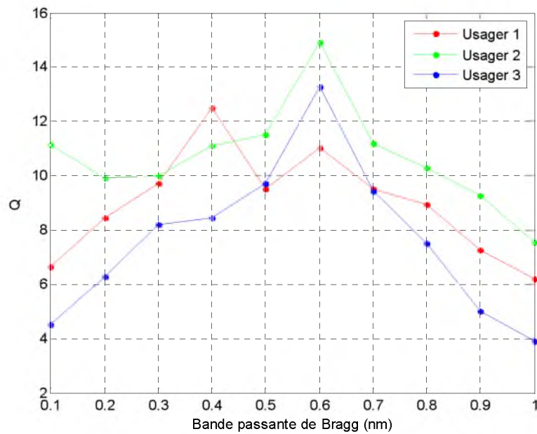
Figure 4.24 Q en fonction de la bande passante des réseaux de Bragg
