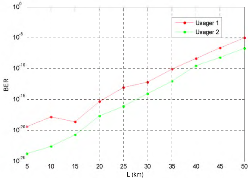
Figure 4.13 BER en fonction de la longueur de la fibre (SMF)
