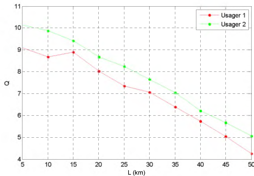
Figure 4.14 Q en fonction de la longueur de la fibre (SMF)
