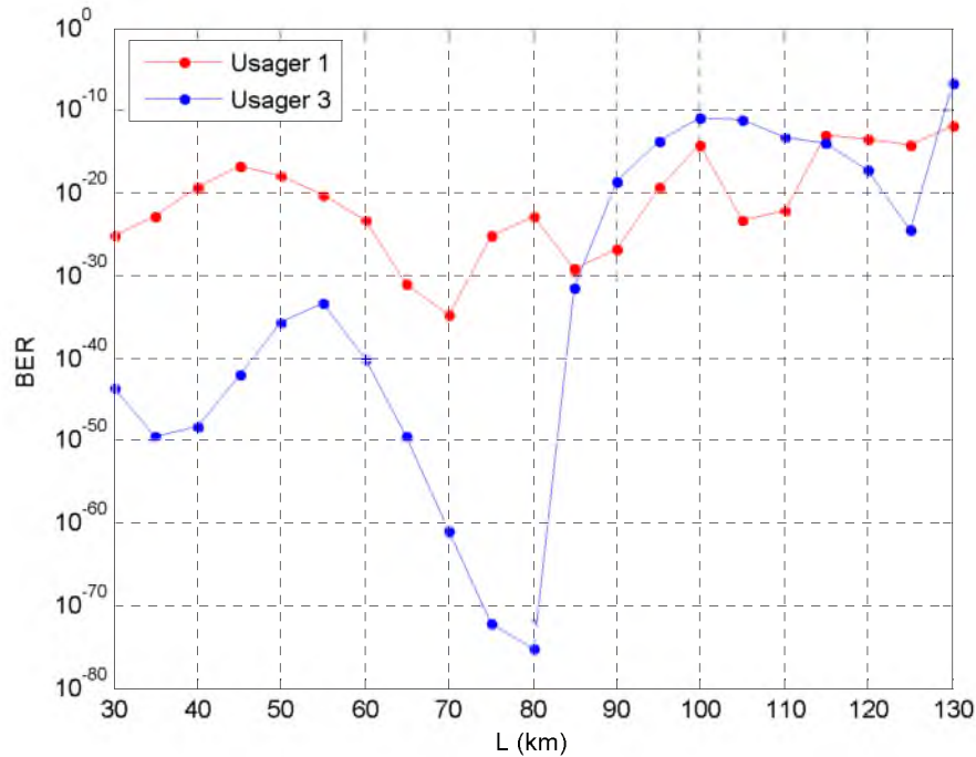
Figure 4.22 BER en fonction de la longueur de la fibre optique (2 éteint, 1 et 3 allumés)
