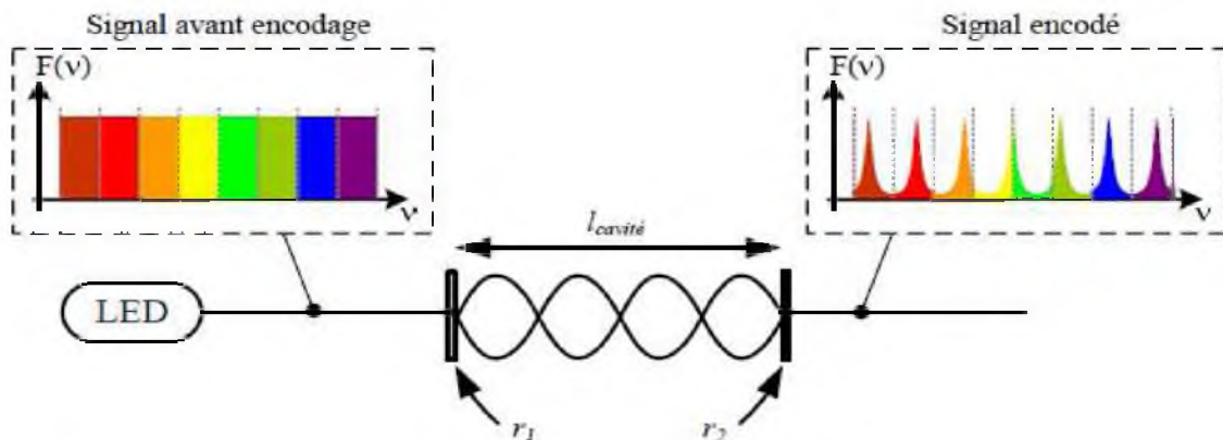
Figure 3.9 Cavité de type Fabry-Perot
