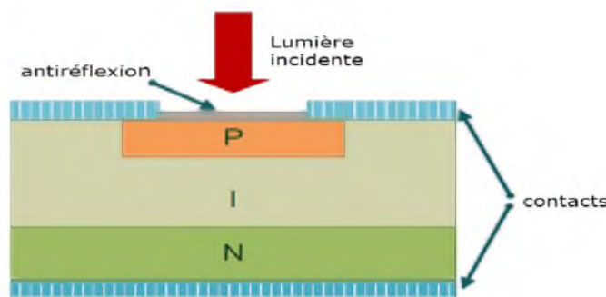
Figure 1.15 Coupe transversale d'une photodiode PIN
