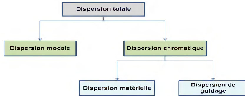
Figure 1.13 Les différents types de dispersion
