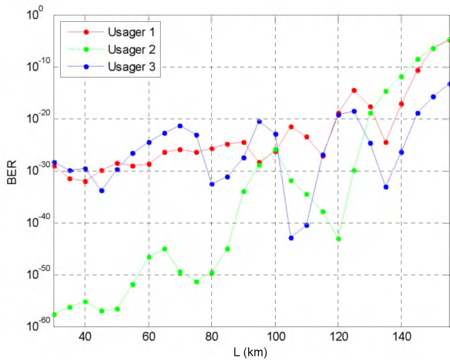
Figure 4.33 BER en fonction de la longueur de la fibre optique
