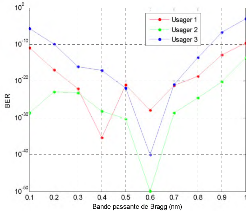
Figure 4.23 BER en fonction de la bande passante des réseaux de Bragg
