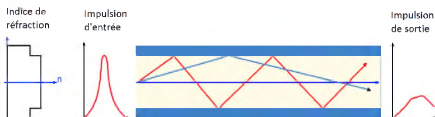
Figure 1.9 Propagation des ondes dans une fibre multimodes à saut d'indice
