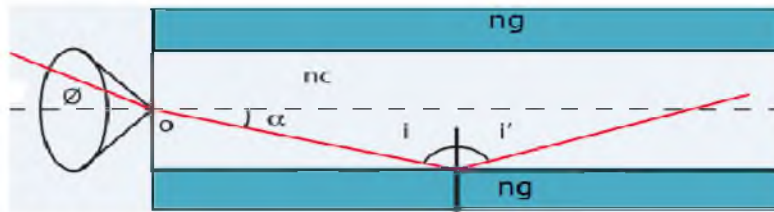
Figure 1.8 Illustration de l'ouverture numérique et du guidage au cœur de la fibre optique
