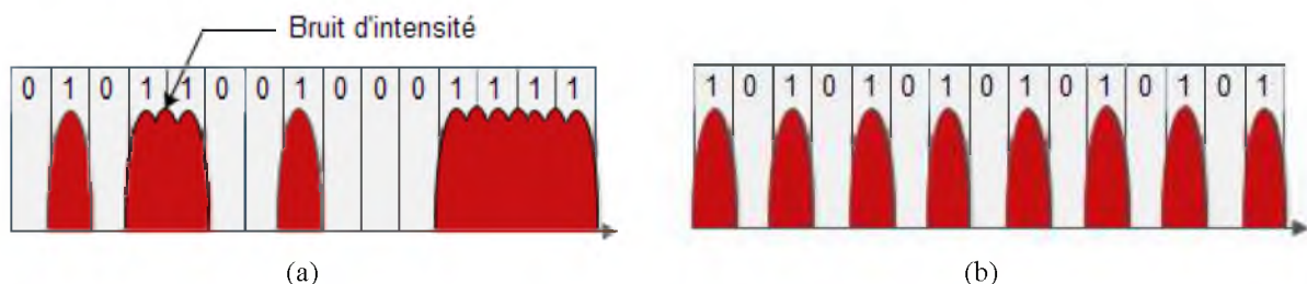
Figure 4.38 Spectres des codes avec des réponses spectrales réelles, (a) pour l'encodeur 1 et (b) pour le code « 1010101010101 »
