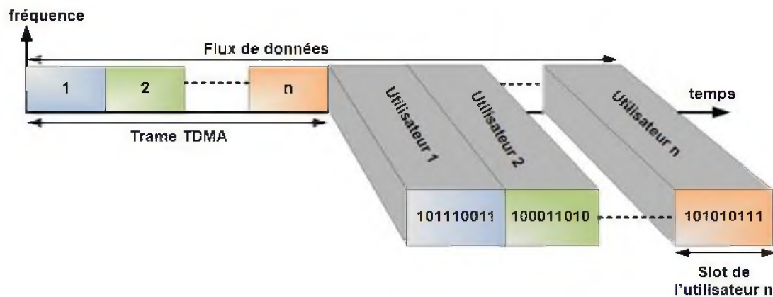
Figure 2.3 L'accès multiple à répartition dans le temps (TDMA)
