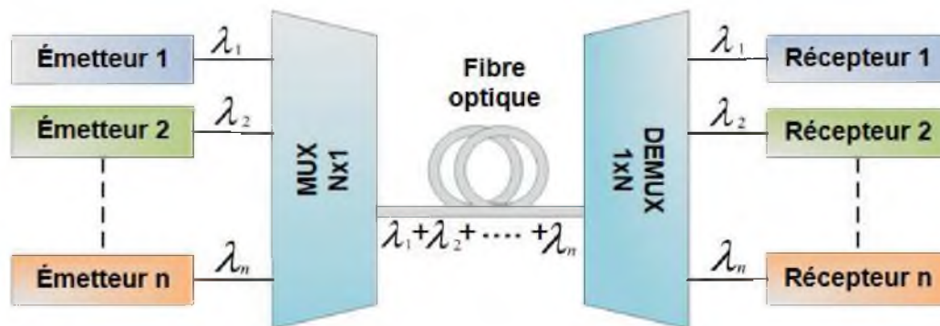
Figure 2.2 L'accès multiple à répartition en longueur d'onde (WDMA)
