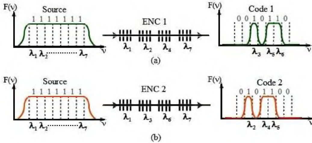
Figure 3.1 Principe de l'encodage spectral SAC-OCDMA (a) pour l'utilisateur désiré avec code 1 ; (b) pour un interférent avec le code 2
