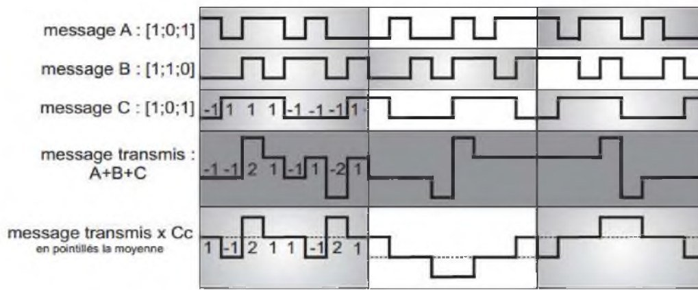
Figure 2.10 Chronogramme de codage et de décodage CDMA
