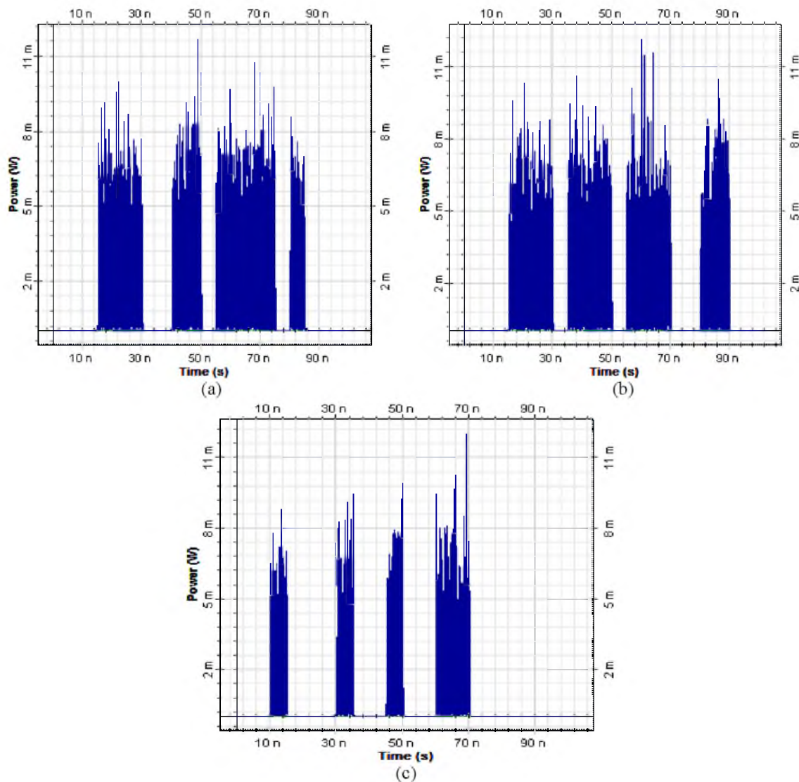
Figure 4.8 Courbes du signal optique à la sortie du deuxième FBG, (a) : premier usager, (b) : deuxième usager, (c) : troisième usager
