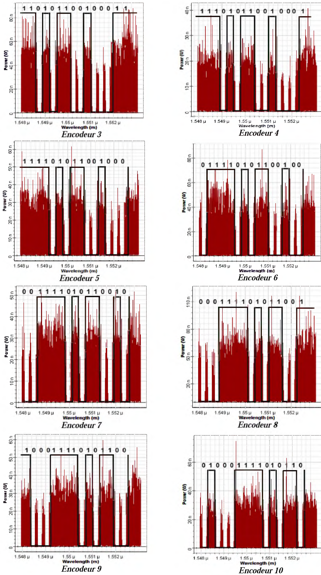
Figure 4.35 Amplitudes spectrales et leurs codes associés des 10 premiers usagers
