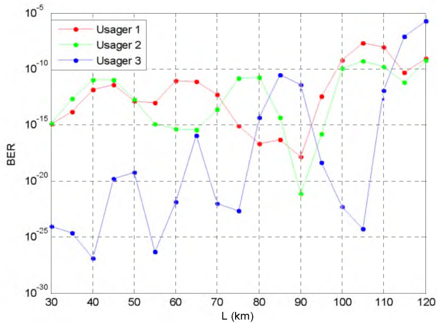
Figure 4.31 BER en fonction de la longueur de la fibre optique pour 3 utilisateurs
