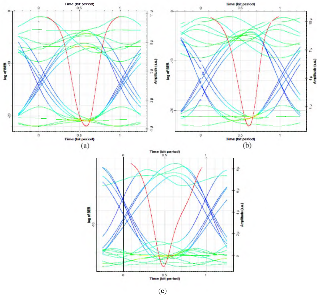
Figure 4.10 Diagrammes de l'œil et BER 10 km, (a) : premier usager, (b) : deuxième usager, (c) : troisième usager
