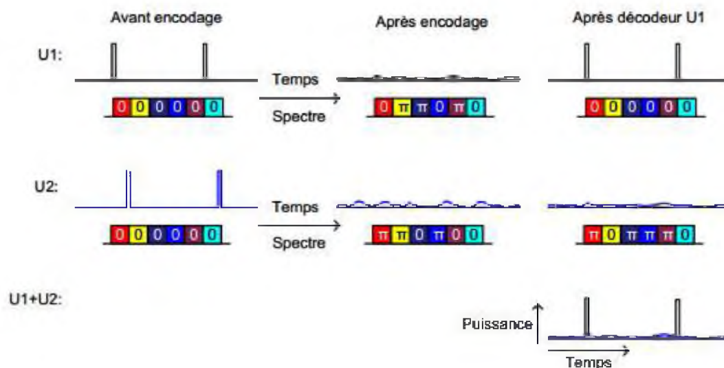
Figure 2.13 Présentation schématique du SPE-OCDMA
