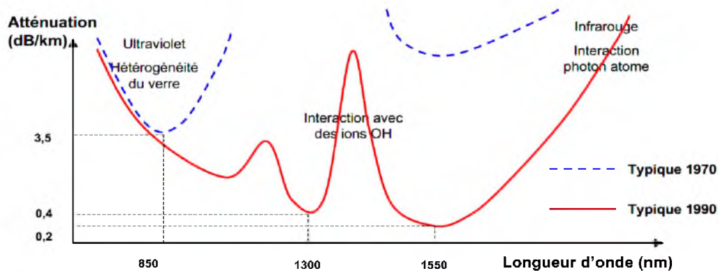
Figure 1.12 Atténuation spectrale d'une fibre en fonction de la longueur d'onde
