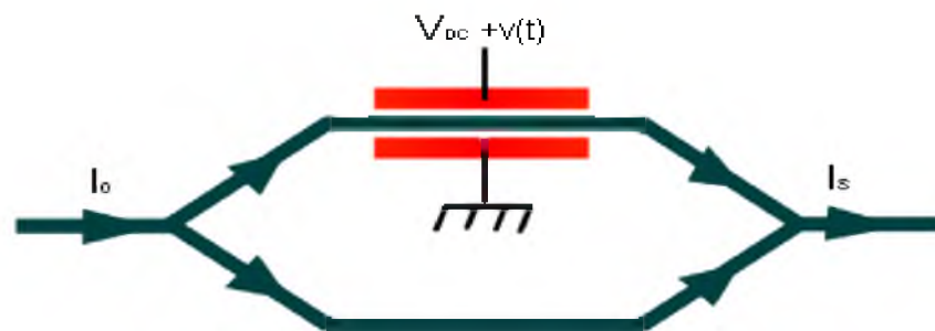
Figure 1.6 Schéma simplifié d'un modulateur de Mach-Zehnder
