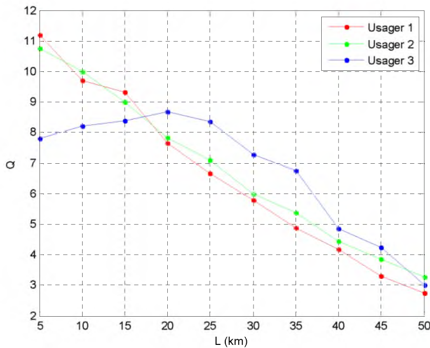
Figure 4.28 Q en fonction de la longueur de la fibre optique pour 3 utilisateurs
