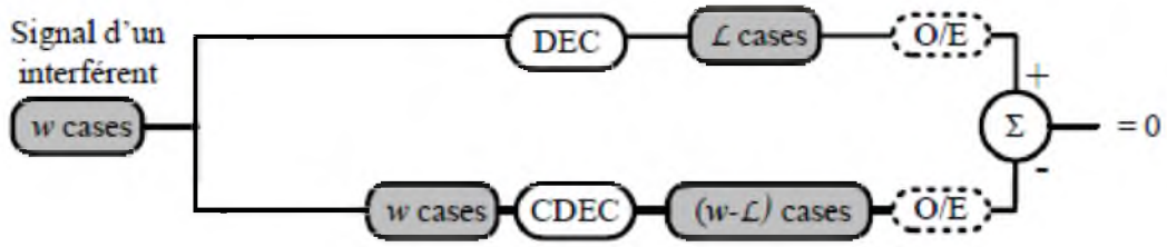
Figure 3.4 Fonctionnement général du système de décodage
