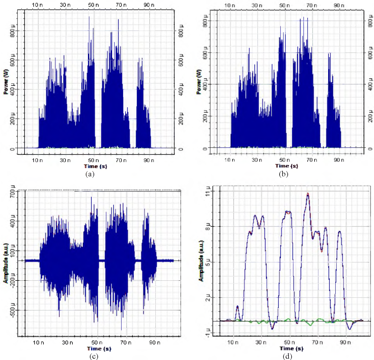
Figure 4.9 (a) : sortie du filtre de décodage H(f) , (b) sortie du filtre de décodage \overline{H}(f) , (c) : photocourant résultant de H(f) et \overline{H}(f) , (d) : version filtré du photocourant résultant
