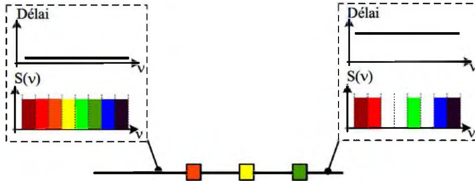
Figure 3.12 Réseaux de Bragg utilisés en transmission pour encodage SAC-OCDMA
