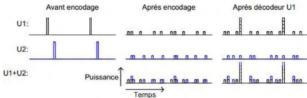
Figure 2.12 Présentation schématique du DS-CDMA
