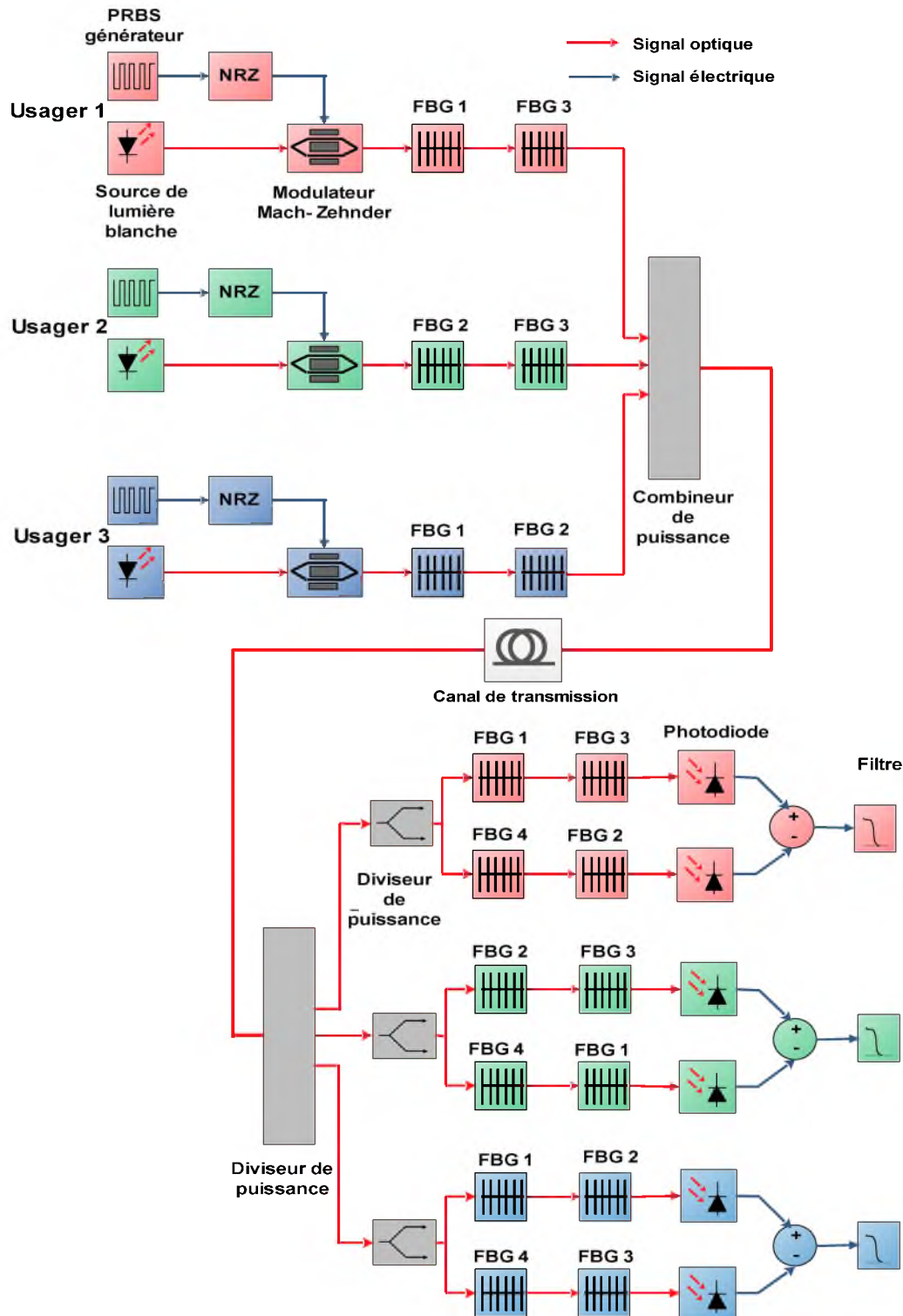
Figure 4.4 Diagramme du système SAC-OCDMA pour 3 usagers
