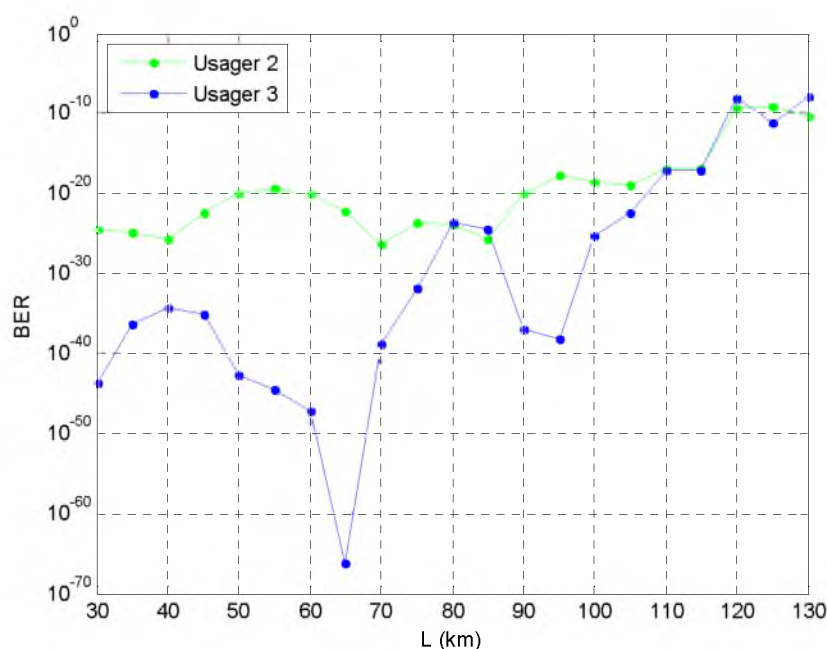
Figure 4.21 BER en fonction de la longueur de la fibre optique (1 éteint, 2 et 3 allumés)
