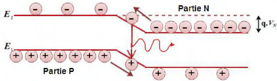
Figure 1.4 Schéma de la jonction P-N dans un laser
