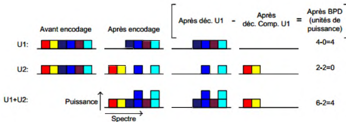
Figure 2.14 Représentation schématique du SAC-OCDMA, chaque couleur représente une case fréquentielle différente
