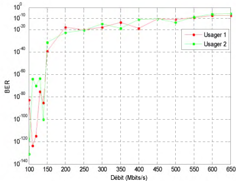
Figure 4.11 BER en fonction du débit binaire
