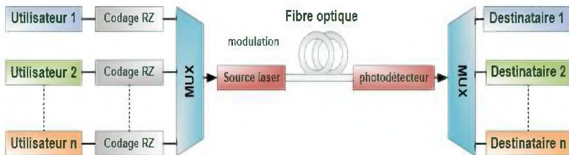
Figure 2.4 L'accès multiple à répartition électrique (ETDMA)
