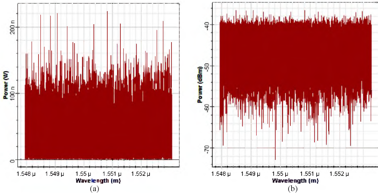
Figure 4.5 Spectre de puissance de la source optique large bande (a) en Watt, (b) en dbm
