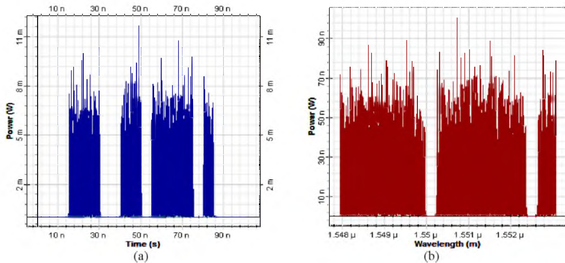
Figure 4.7 Les courbes de l'encodage du premier usager, (a) domaine temporel, (b) domaine spectral
