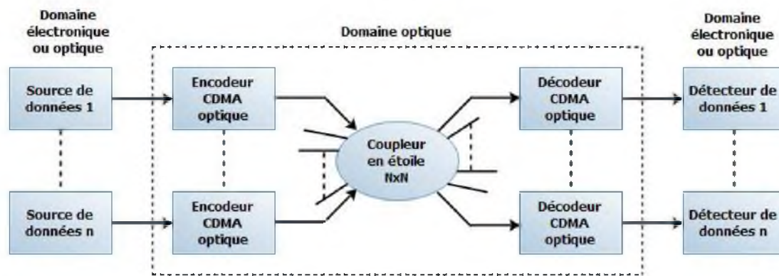
Figure 2.11 OCDMA avec émetteurs et récepteurs optiques en configuration en étoile
