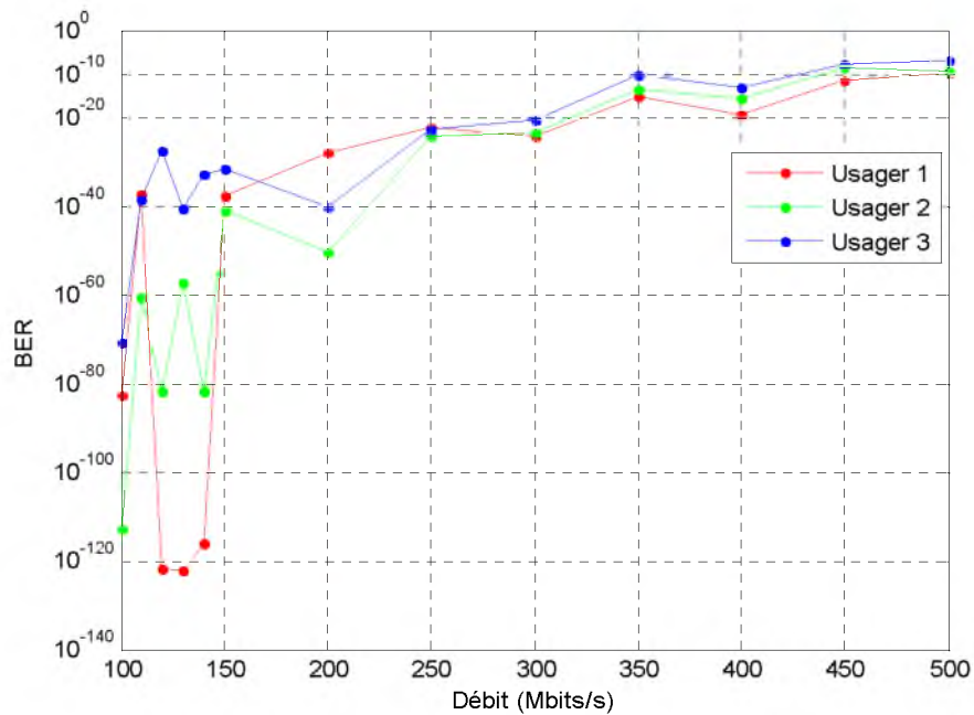
Figure 4.30 BER en fonction du débit binaire
