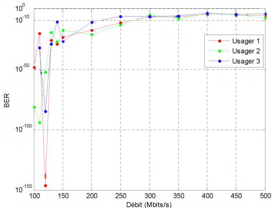
Figure 4.32 BER en fonction du débit binaire
