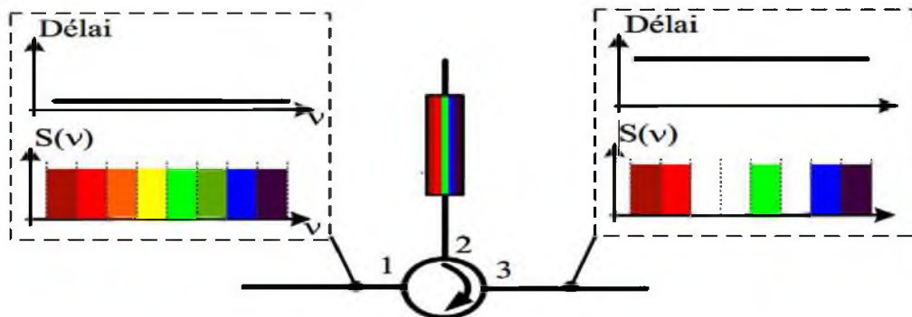
Figure 3.11 Réseaux de Bragg superposés pour encodage SAC-OCDMA
