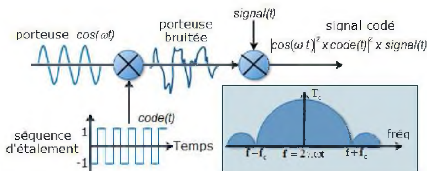
Figure 2.6 Encodage d'un système DS-SS et spectre du signal étalé
