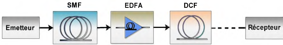
Figure 1.16 Schéma d'une liaison optique avec compensation et gestion d'atténuation
