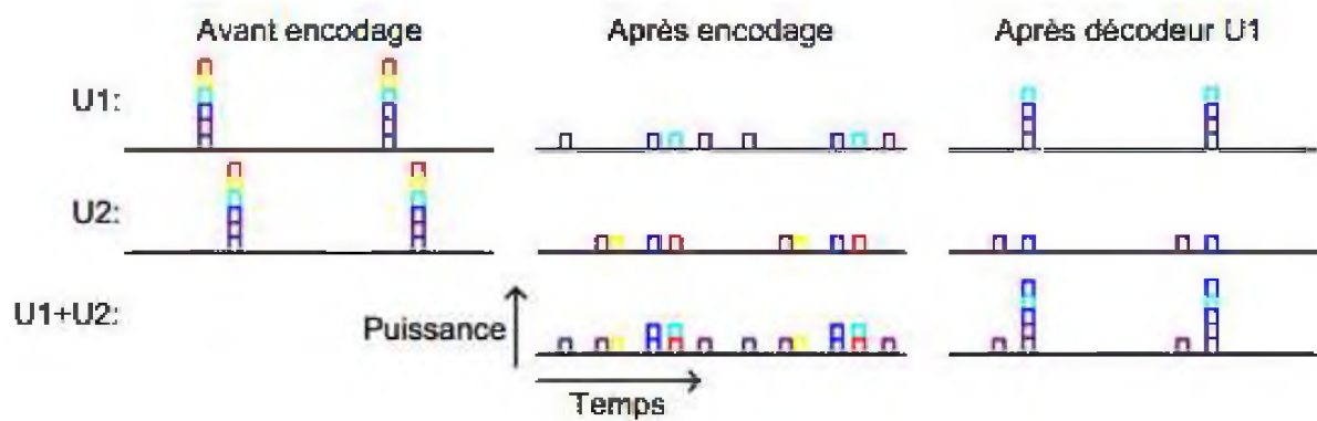
Figure 2.16 Représentation schématique d'un système (\lambda/t) OCDMA
