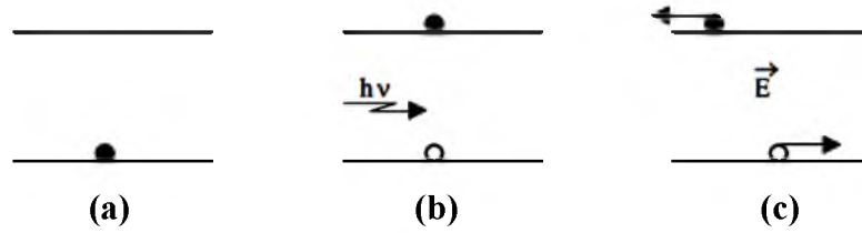
Figure 1.14 Niveaux d'énergie
