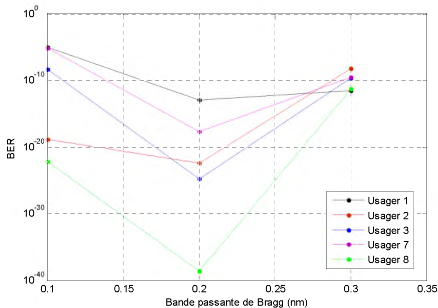
Figure 4.39 BER en fonction de la Bande passante de Bragg
