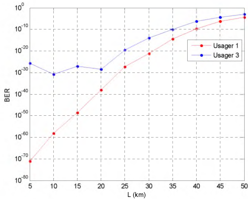
Figure 4.17 BER en fonction de L (2 éteint, 1 et 3 allumés)
