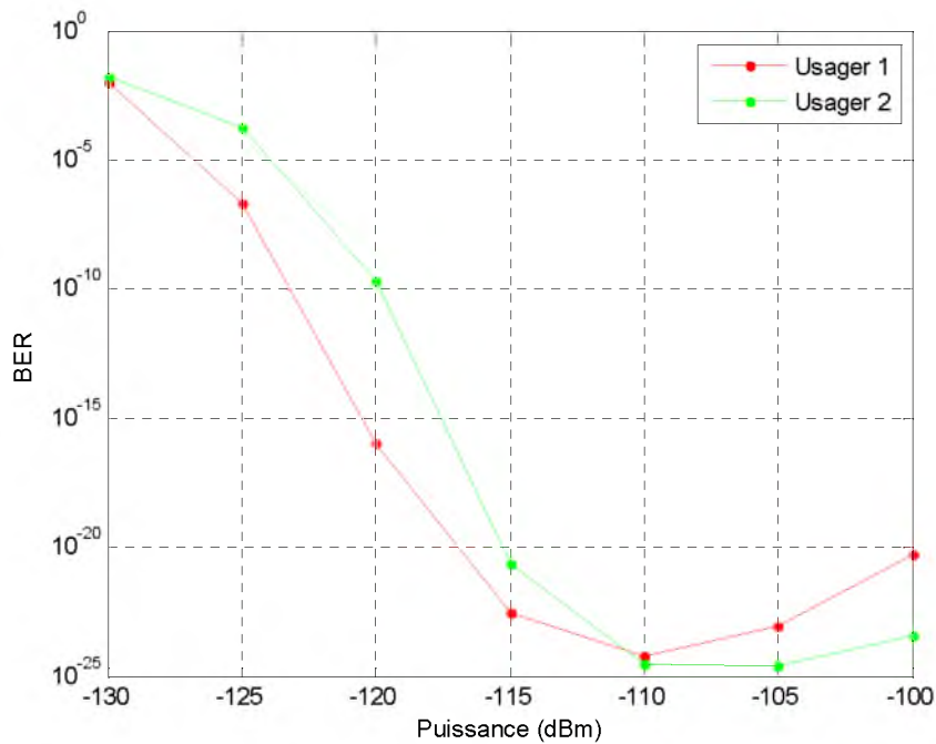
Figure 4.19 BER en fonction de la puissance des sources optiques
