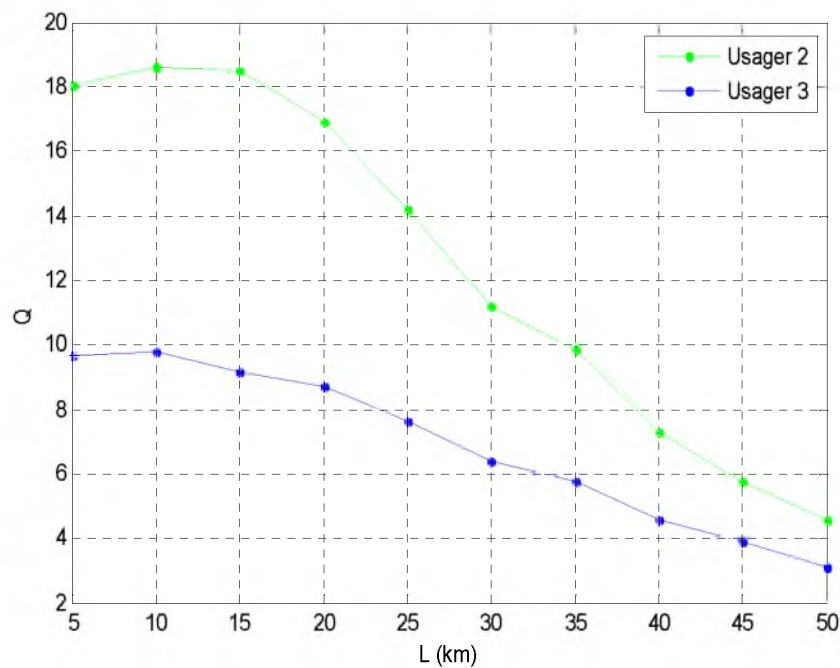
Figure 4.16 Q en fonction de L (1 éteint, 2 et 3 allumés)
