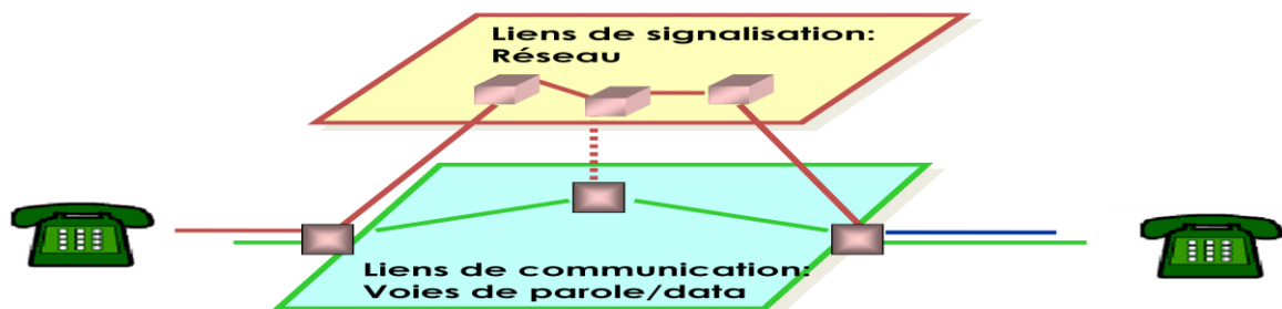
Figure I.9: architecture du réseau SS7
