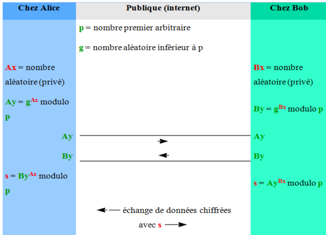
Figure II.4 : échange de clés de Diffie et Hellman
