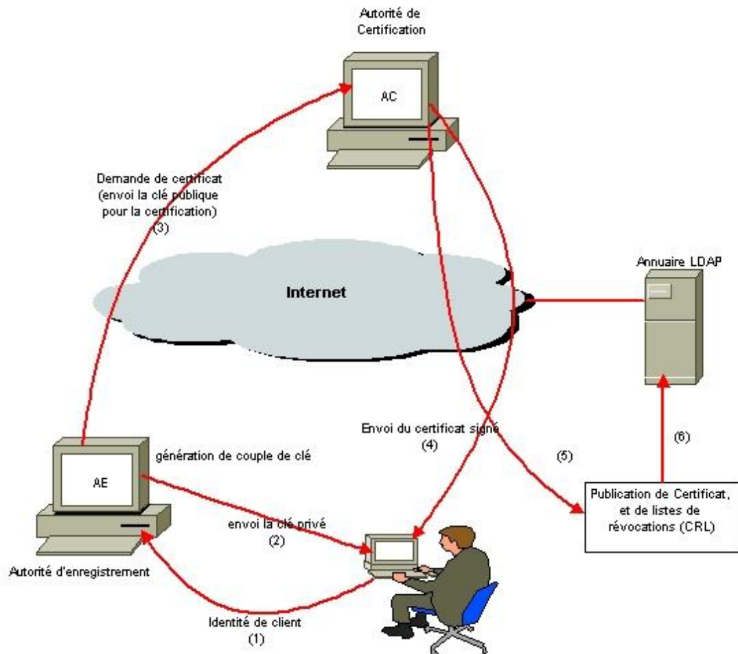
Figure II.7: Organisation d'une PKI
