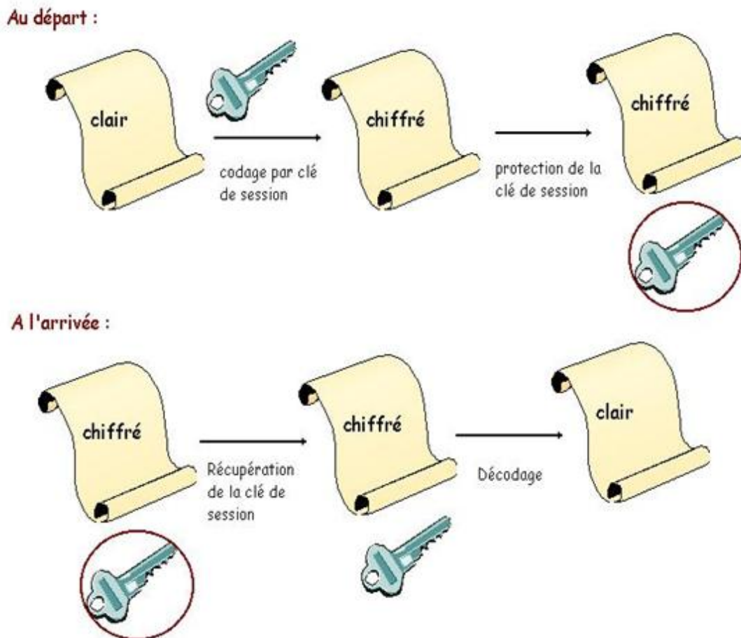
Figure II.9: Principe de chiffrement du PGP
