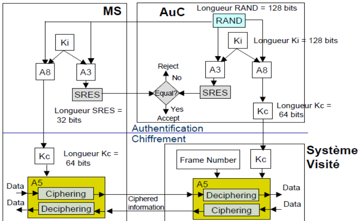
Figure I.6: Sécurité GSM
