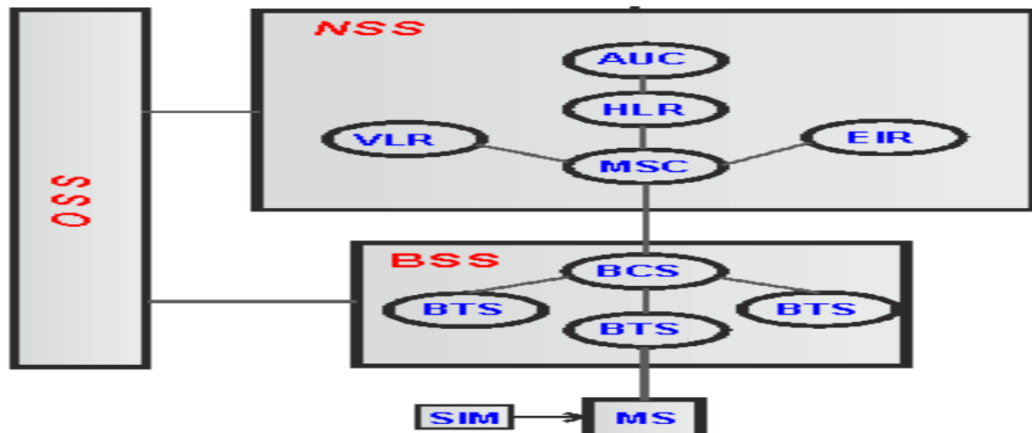
Figure I.1 : architecture de réseau GSM
