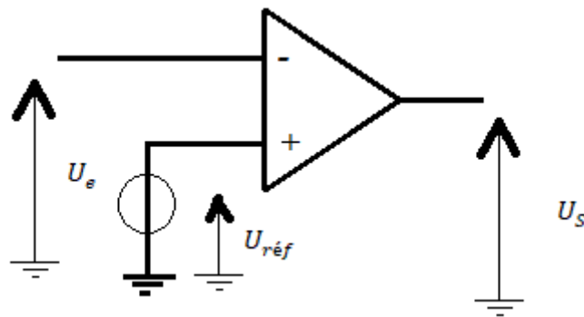
Figure 2.27: Comparateur inverseur
