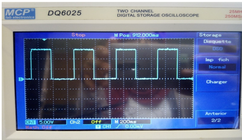
Figure 3.19 : Point M : la sortie de l'oscillateur
