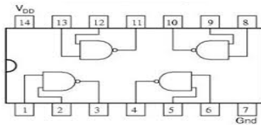
Figure 2.5: Circuit intégré CD4011
