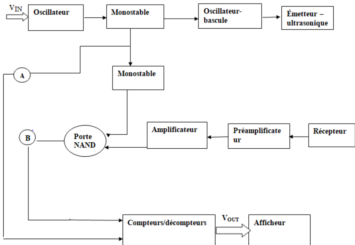
Figure 2.1: Schéma bloc
