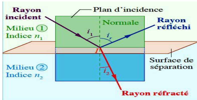
Figure 1.7: Phénomène de réflexion et réfraction des ondes ultrasonores
