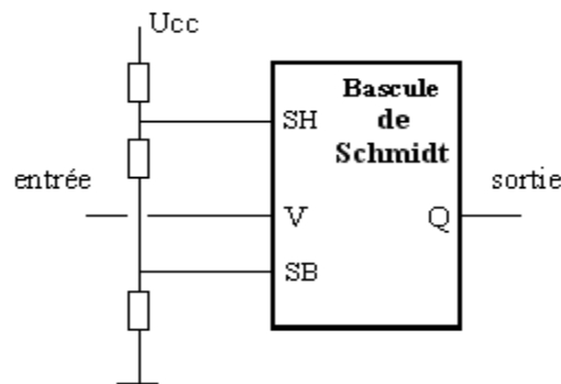
Figure 2.18: Symbole du Trigger de Schmitt
