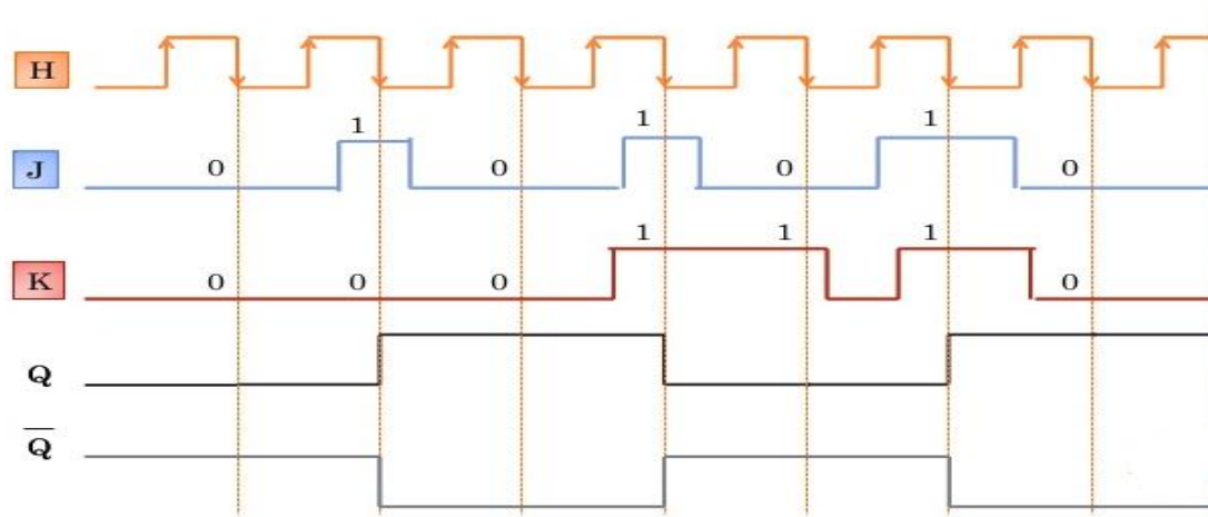
Figure 19 : Chronogramme
