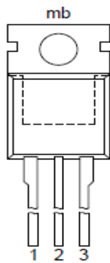
Figure 26 : Brochage du triac
