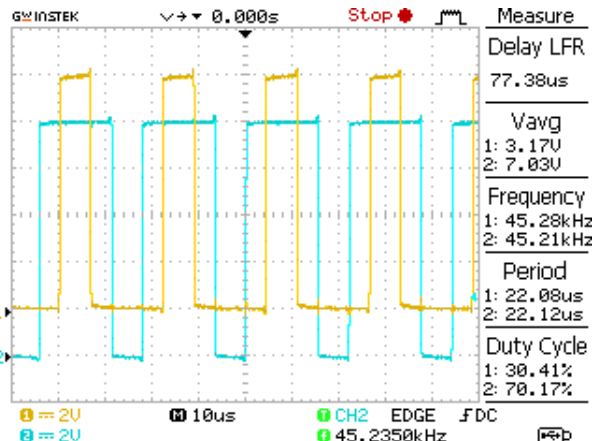
Figure 4-2.b : Forme de la PWM
