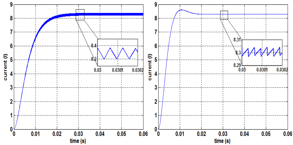
(a) Boost classique
