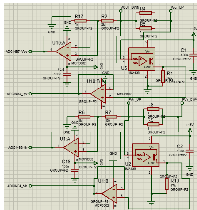
Figure 4-4 : Schéma de l'acquisition des données
