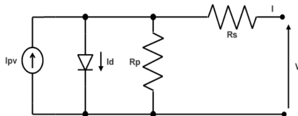
Figure02-1 : modèle équivalent d'une cellule photovoltaïque
