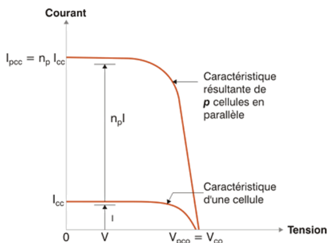
Figure 1-6 : Association des cellules en parallèle
