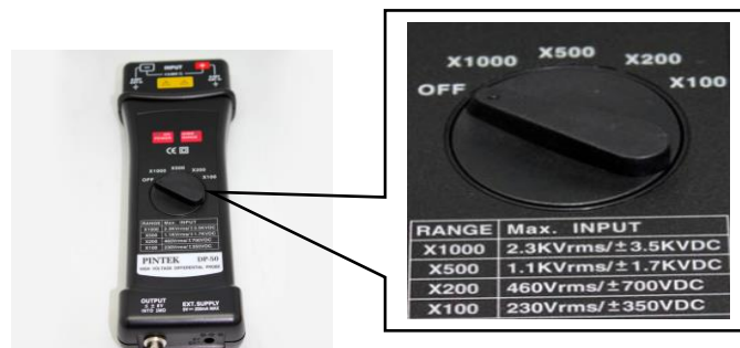
Figure 04-6 : Sonde Différentielle de tension DP-50
