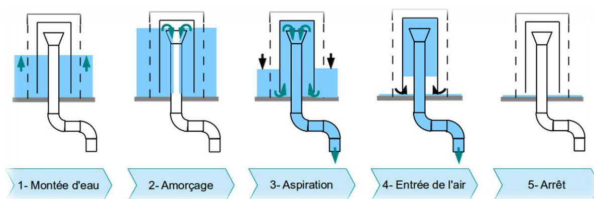
Figure 1.10 : Fonctionnement le siphon-cloche en aquaponie
