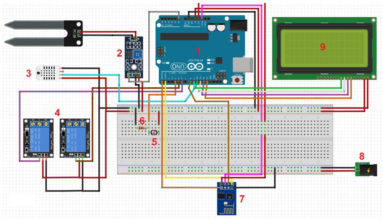
Figure 25 : Montage du système final
