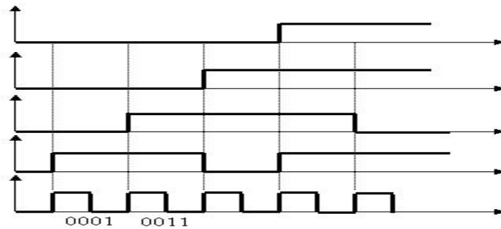
Figure 17 : Signaux numériques
