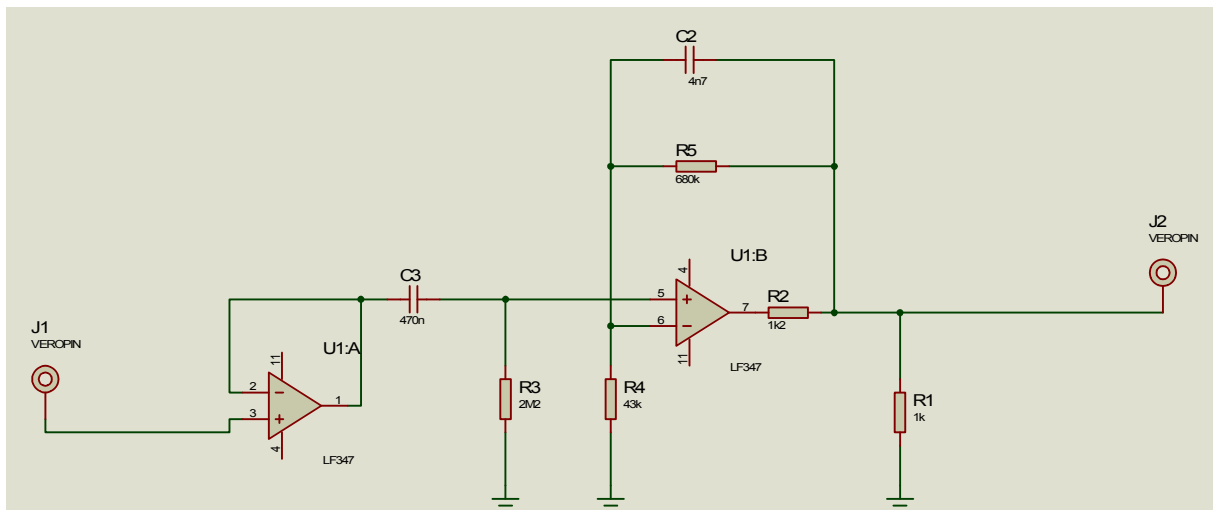
Figure II.9 : Circuit de filtrage
