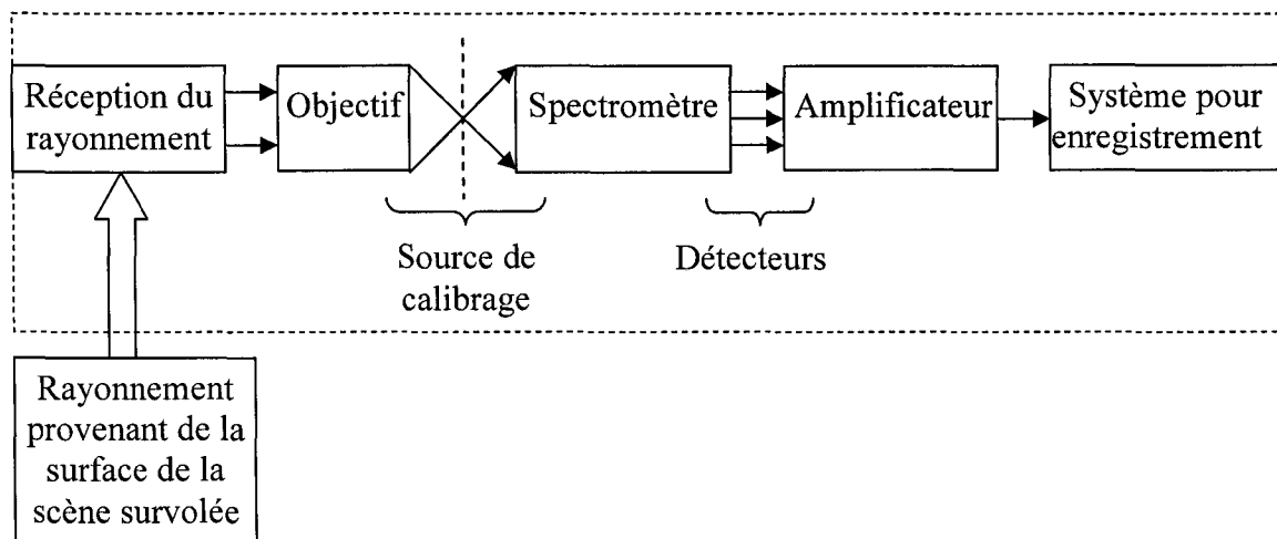
Figure 20 Schéma général d'un capteur numérique [74]
