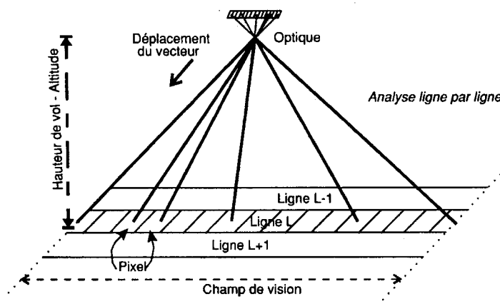
Figure 22 Schéma de principe d'un système à barrettes
