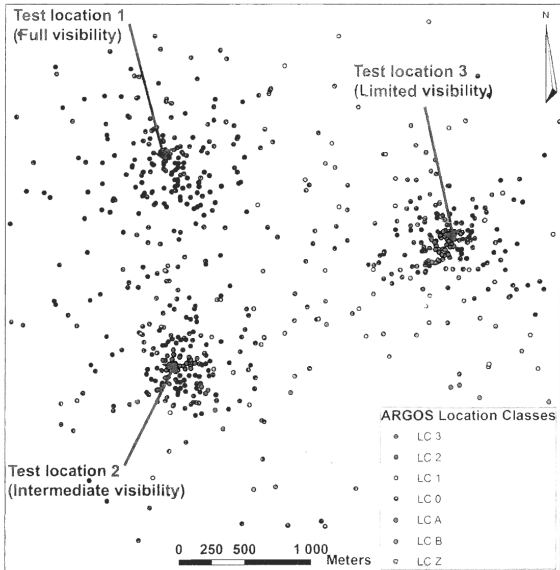
Figure 1.6 Emplacement relatif des trois positions-test utilisées pour estimer l'erreur de localisation de 12 colliers Argos suivant le pourcentage de couverture céleste cachée par le relief. Les courbes représentent les courbes de niveau (espacées de 10 m) et les zones grisées sont des plans d'eau. Test 1 : bonne [66%-100%]; Test 2 : intermédiaire [33%-66%]; Test 3 : limitée [0%-33%]. L'extrémité de chaque flèche indique l'emplacement de la position-test estimée par GPS.
