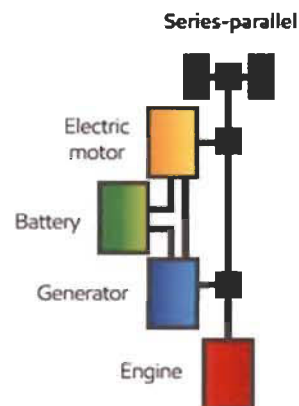
Figure 2-10 : Configuration série-parallèle [40].
