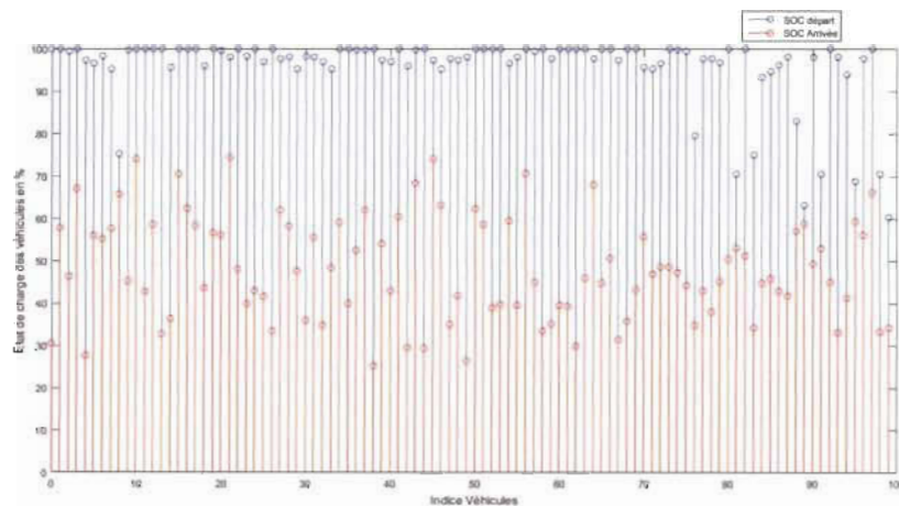
Figure 5-14 : États de charge, 100 Model S, arrivée-départ.
