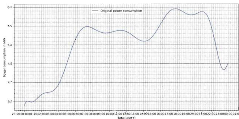
Figure 5-15 : Appels de puissance, 23 février 2015
