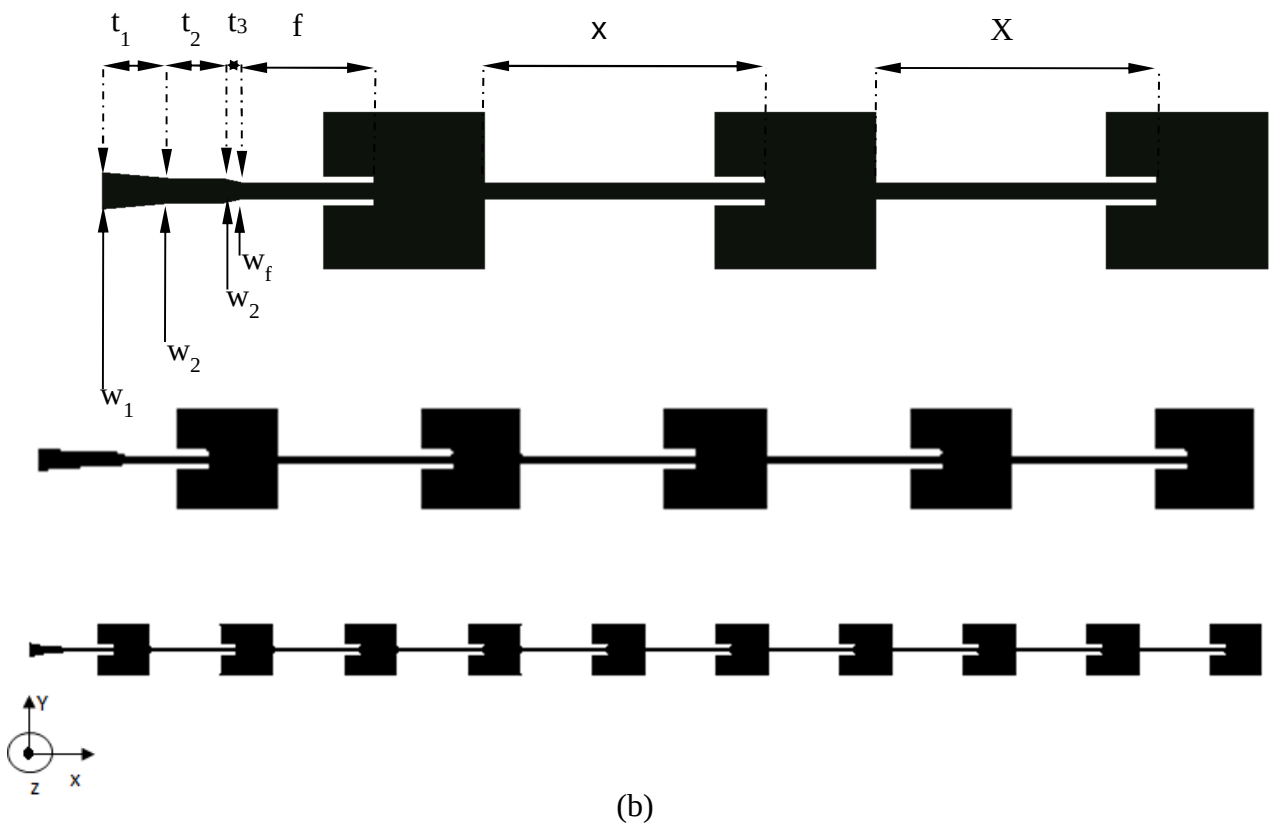
Figure III. 5. Les masques des réseaux d'antennes fonctionnant à 2.44 GHz pour applications Bluetooth. (a). Cinq éléments rayonnants, (b). Dix éléments rayonnants.
