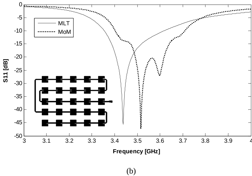
Figure III. 40. Coefficients de réflexions obtenus par le circuit électrique et le simulateur Momentum (a). Réseau d'antennes à 5 \times 2 éléments, (b). Réseau d'antennes à 10 \times 5 éléments.
