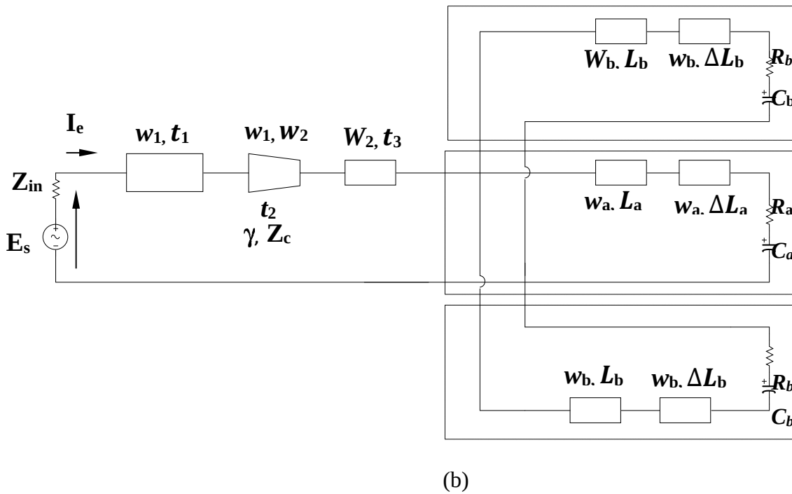
Figure III. 21. (a). Masque de l'antenne fonctionnant à 1.95 GHz pour système UMTS. (b) Schéma électrique équivalent de l'antenne UMTS proposée. Les paramètres de l'antenne sont: L_a = 20.08 \text{ mm} , W_a = 7.37 \text{ mm} , L_b = 10.95 \text{ mm} , W_b = 15.97 \text{ mm} , L_c = 10.95 \text{ mm} , W_c = 15.97 \text{ mm} , W_f = 3.04 \text{ mm} et y = 45.95 \text{ mm} .
