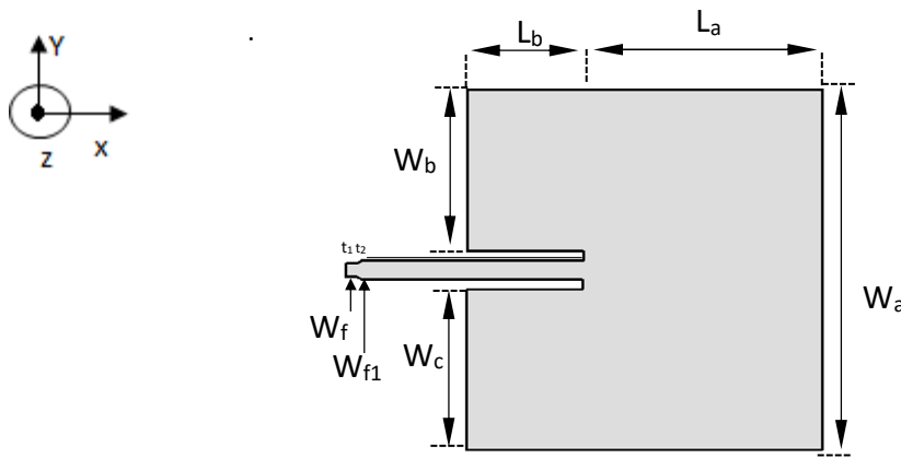
Figure IV. 5. Masque de l'antenne fonctionnant à 1.8 GHz pour système GSM/LTE. Les paramètres de l'antenne sont : L_a = 20.08\text{ mm} , W_a = 57.11\text{ mm} , L_b = 18.35\text{ mm} , L_a = 37.58\text{ mm} , W_b = 25.64\text{ mm} , W_c = 25.64\text{ mm} , W_f = 2.09\text{ mm} , W_{f1} = 3.43\text{ mm} , y = 45.95\text{ mm} , t_1 = 2.14\text{ mm} , t_2 = 34.17\text{ mm} .
