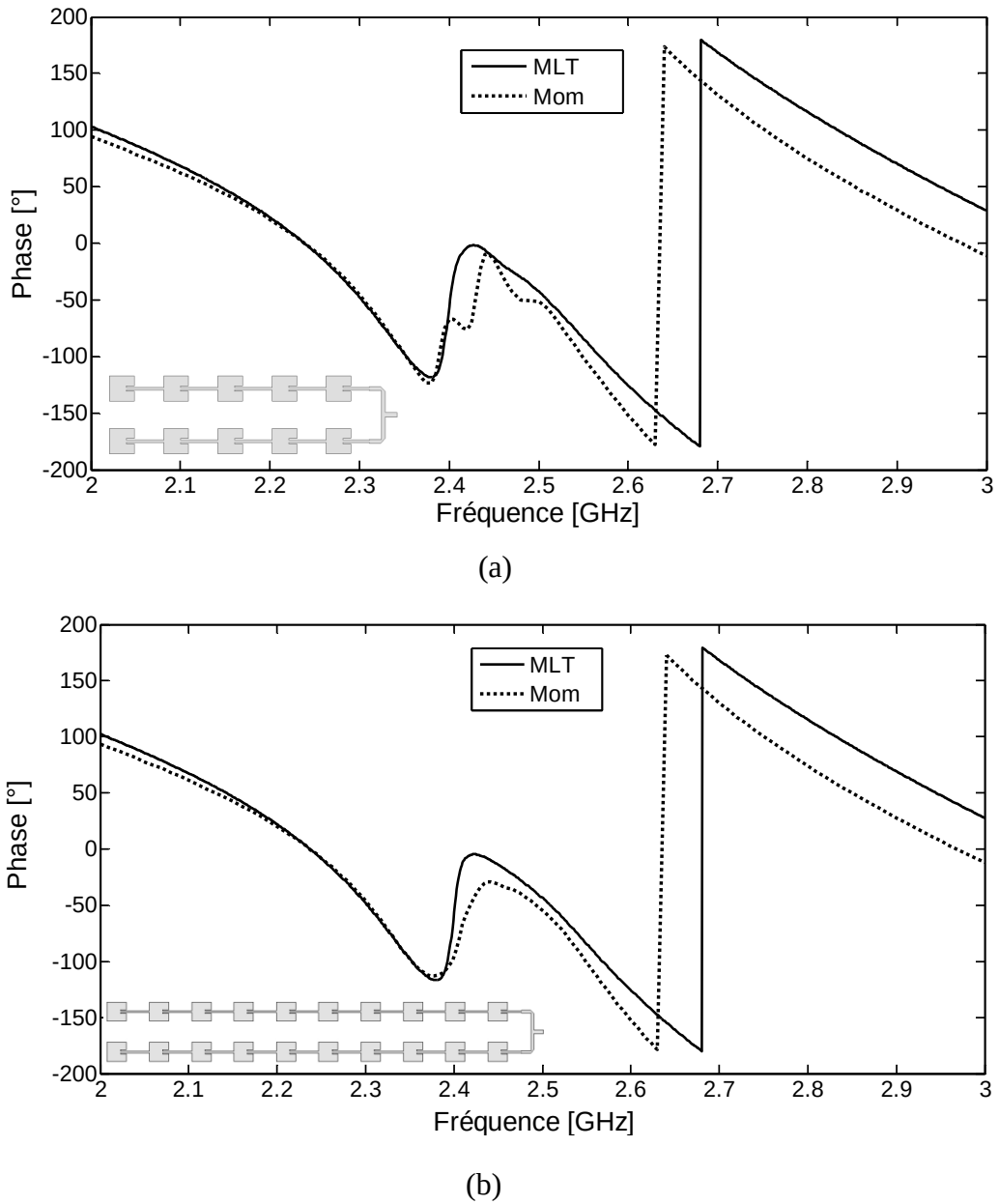
Figure III. 19. Phases réfléchies à l'entrée des réseaux obtenues par simulations issues du modèle électrique équivalent et sous Momentum. (a). Réseau d'antennes 5 \times 2 . (b). Réseau d'antennes 10 \times 2 .
