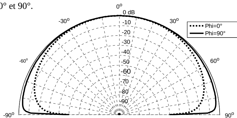
Figure III. 24. Diagramme de rayonnement en 2D de l'antenne seule opérant à la fréquence 1.95 GHz. Simulation obtenu par le simulateur Momentum.
