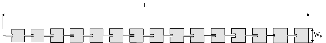
Figure IV. 14. Masque du réseau d'antennes log-périodique à quinze éléments conçu pour application GSM/LTE, les paramètres du réseau d'antennes sont : L = 1265.89 mm, 57.50 mm.
