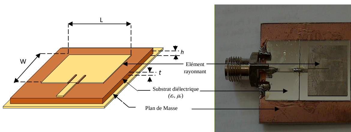
Figure I. 1. Structure d'une antenne imprimée [24].
