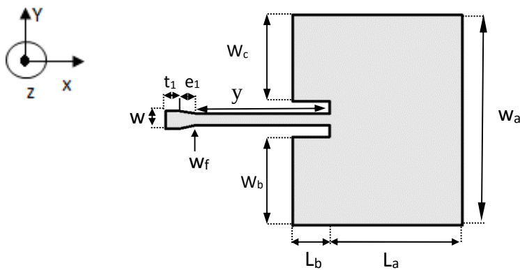
Figure IV. 1. Masque de l'antenne fonctionnant à 1.8 GHz pour système GSM/LTE. Les paramètres de l'antenne sont : L_a = 31.41 \text{ mm} , W_a = 49.66 \text{ mm} , L_b = 8.77 \text{ mm} , W_b = 20.52 \text{ mm} , L_c = 8.77 \text{ mm} , W_c = 20.52 \text{ mm} , W_f = 2.56 \text{ mm} , W = 3.94 \text{ mm} , t_1 = 1.55 \text{ mm} , e_1 = 6.80 et y = 39.17 .
