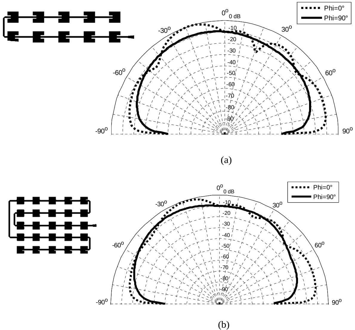
Figure III. 41. Diagramme de rayonnement simulé à la fréquence 3.50 GHz. (a). Réseau à 5×2 éléments rayonnants, (b). Réseau plan de 5×5 éléments rayonnants.
