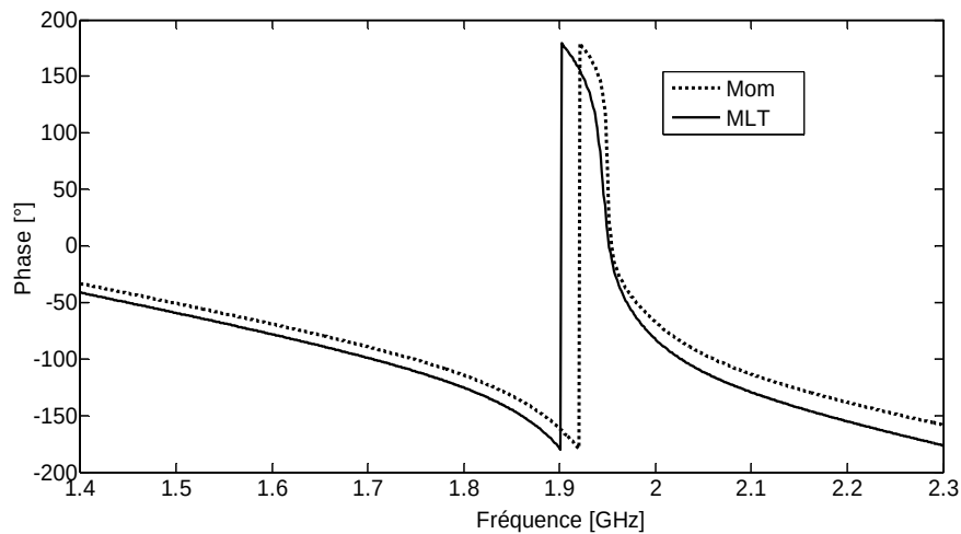
Figure III. 23. Phase réfléchi à l'entrée de l'antenne pour application UMTS présentée sur la figure III. 21. (a).
