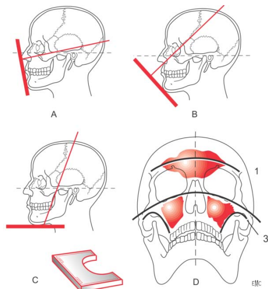
Figure 21 : Incidences radiographiques.
